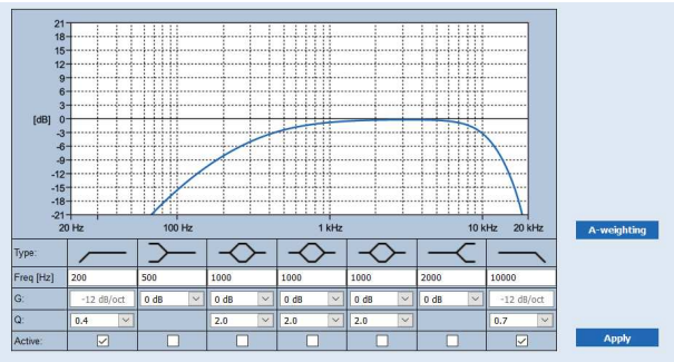
F：频率，G：增益，Q：品质因数
