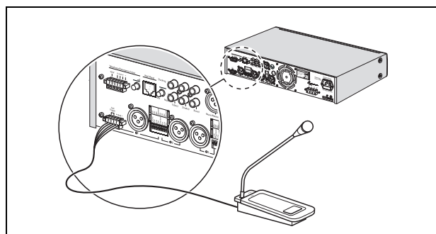
rys. 4.3: Połączenie mikrofonu przy pomocy złącza Euro i wejścia wyzwalającego.
