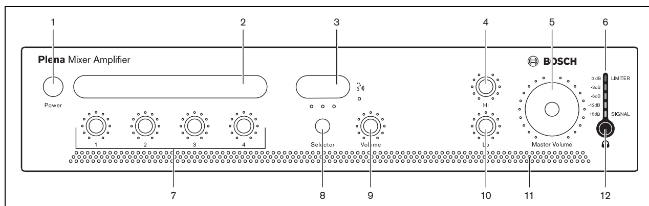
rys. 2.2: Płyta przednia
