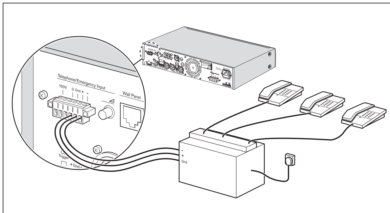
rys. 4.6: Podłączanie alarmowych linii telefonicznych
