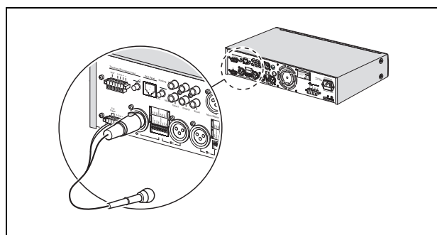
rys. 4.2: Połączenie mikrofonu przy pomocy złącza XLR i wtyku wyzwalającego.
