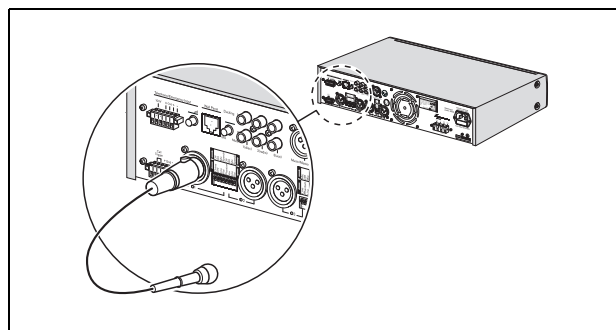
rys. 4.1: Połączenie mikrofonu wyłącznie przy pomocy złącza XLR.
