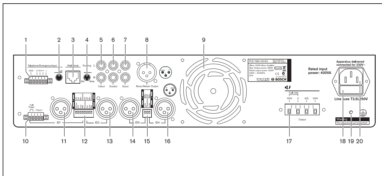
rys. 2.3: Płyta tylna
