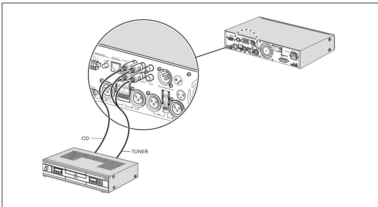
rys. 4.7: Podłączanie źródeł sygnału muzycznego
