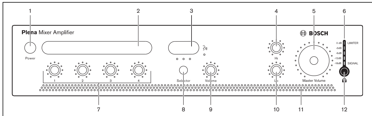
figure 5.1: Panneau avant
