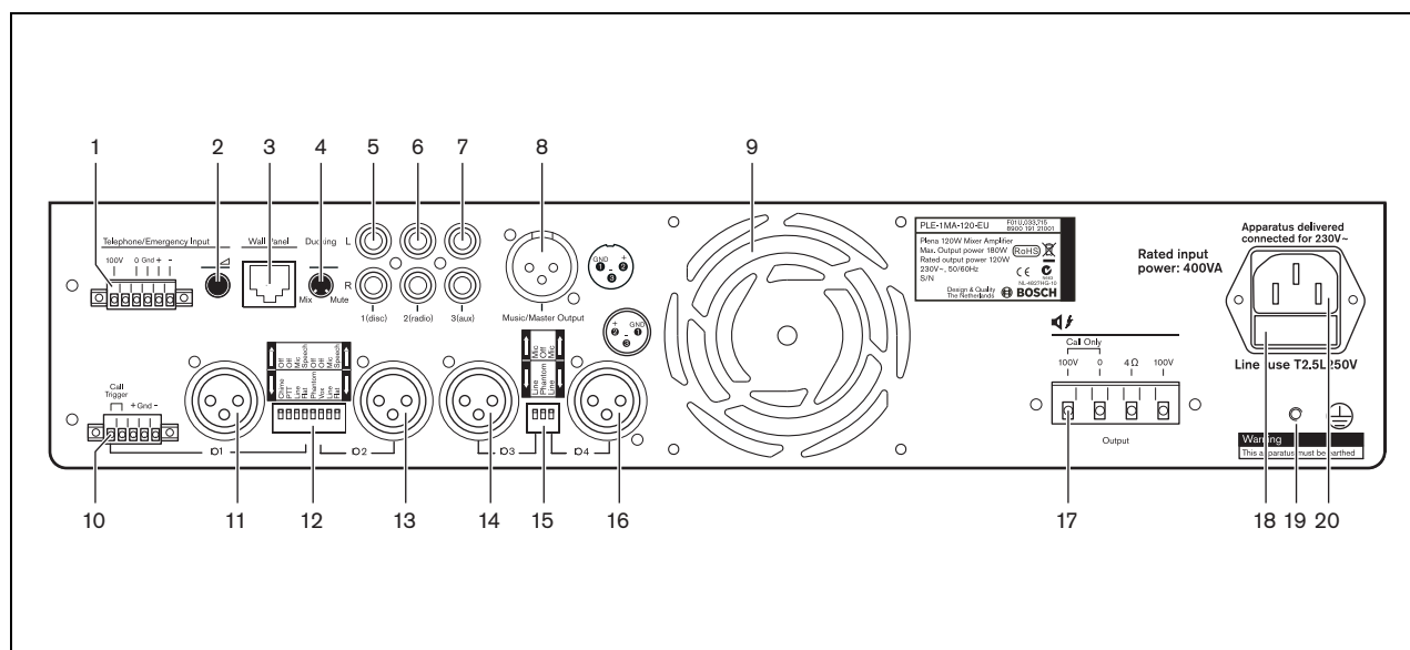
figure 2.3: Panneau arrière
