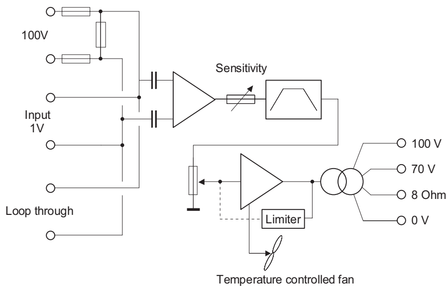
figur 2.1: Skjematisk oversikt over Plena Kraftforsterker
