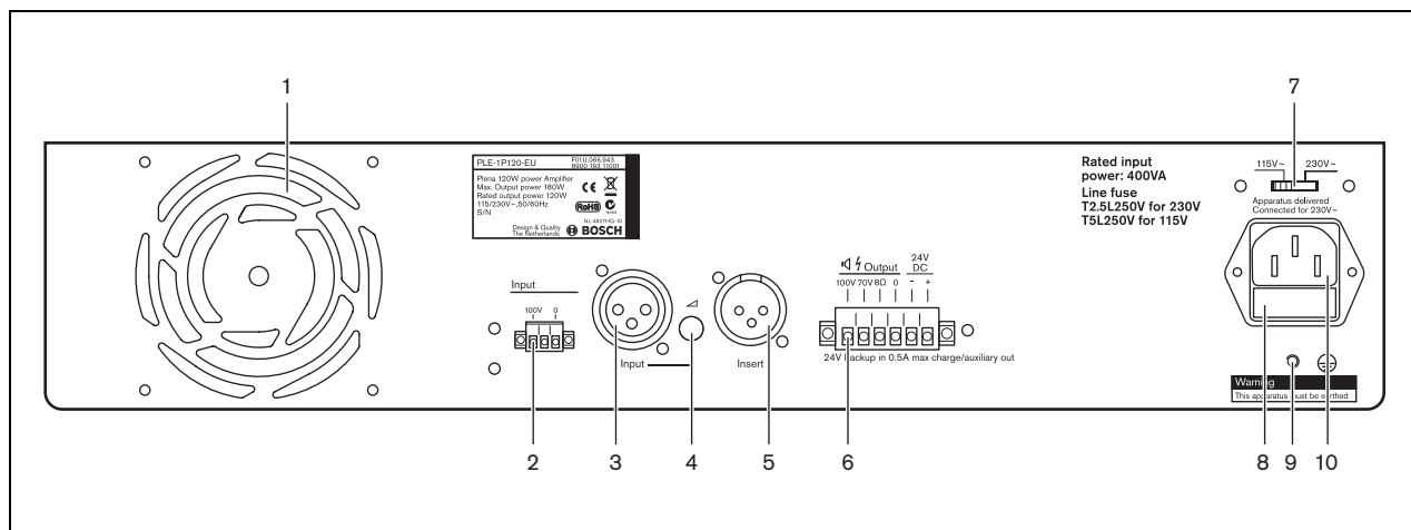
Abbildung 2.3: Rückseite
