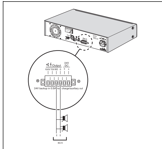
Abbildung 4.4: Anschluss der Lautsprecher
