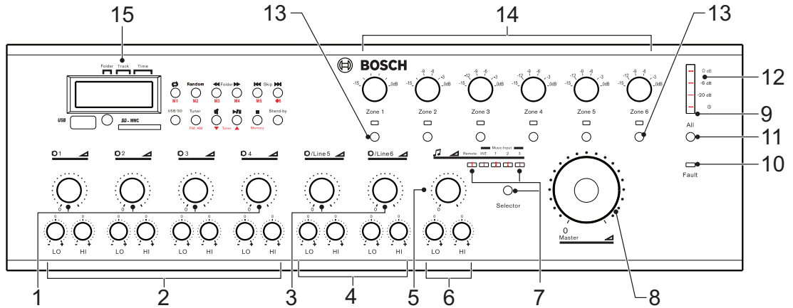
그림 8.1: 전면 패널
