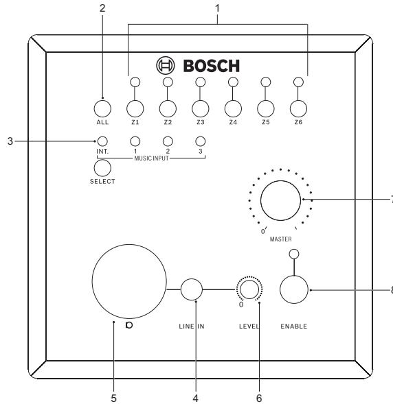
그림 6.5: 벽면 패널 연결
