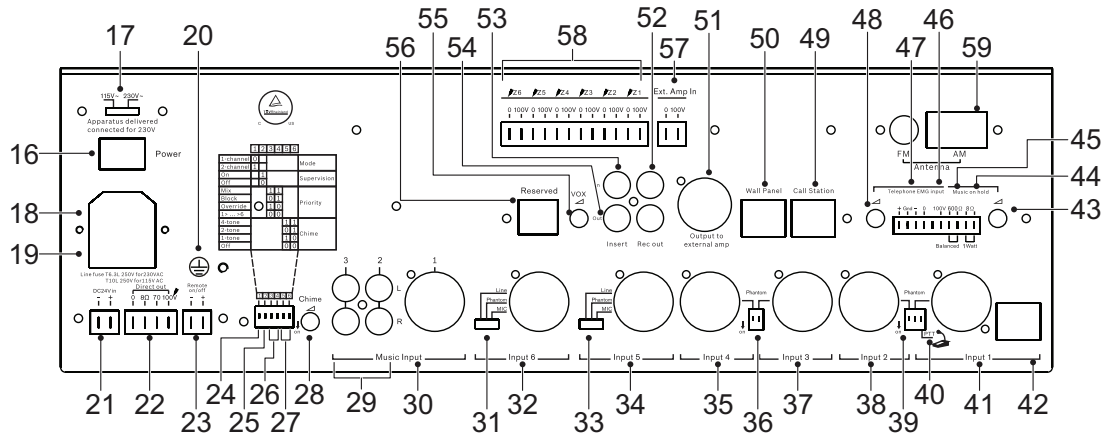
그림 7.1: 후면 패널
