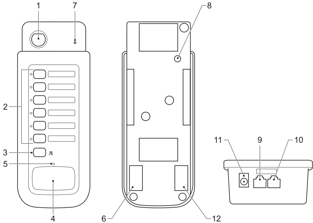
그림 6.4: PLN-6CS 콜 스테이션 연결
