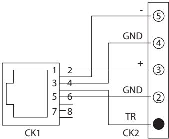
그림 6.3: 마이크 어댑터 커넥터 레이아웃
