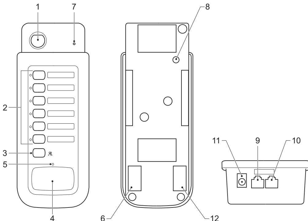
그림 7.2: 콜 스테이션
