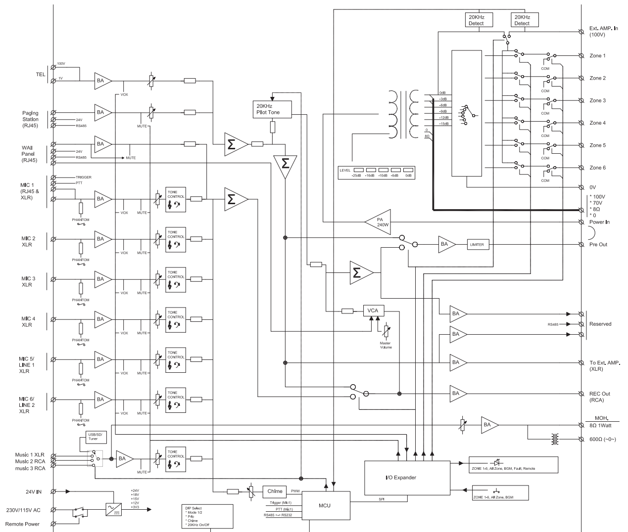
그림 3.1: 올인원 장치 블록 다이어그램
