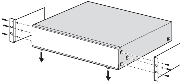
그림 5.1: 19인치 랙에 장치 설치
