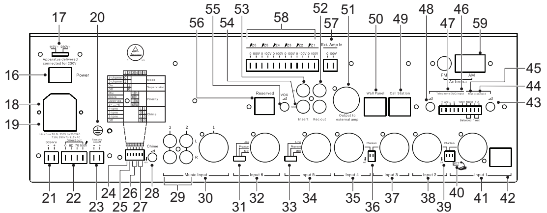
그림 8.2: 후면 패널
