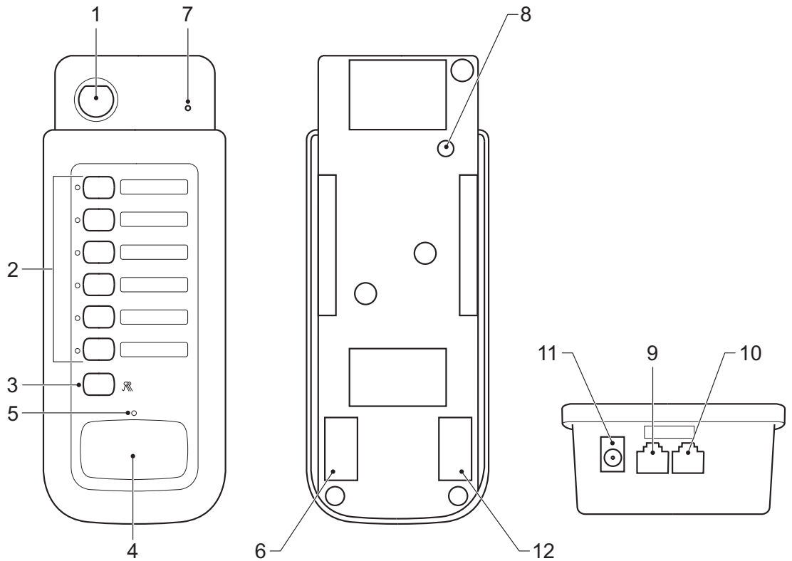
그림 8.5: PLN-6CS 콜 스테이션 기능
