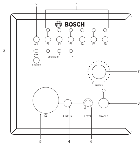
그림 7.3: 벽면 패널 구성
