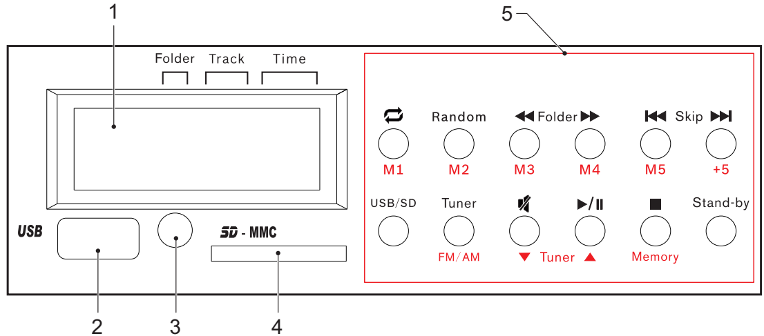
그림 8.3: 오디오 소스 모듈
