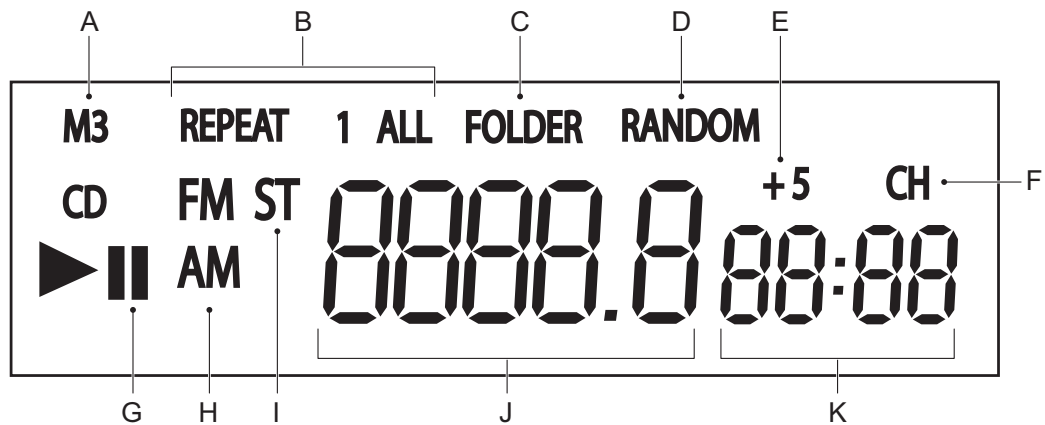
그림 8.4: SD/USB/튜너 LCD 디스플레이 (1)
