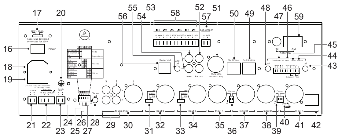
Figura 8.2: Pannello posteriore
