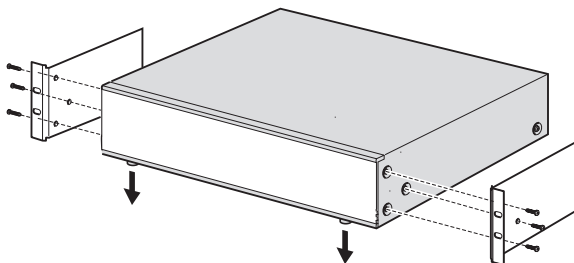
Figura 5.1: Installazione dell'unità in rack da 19 pollici
