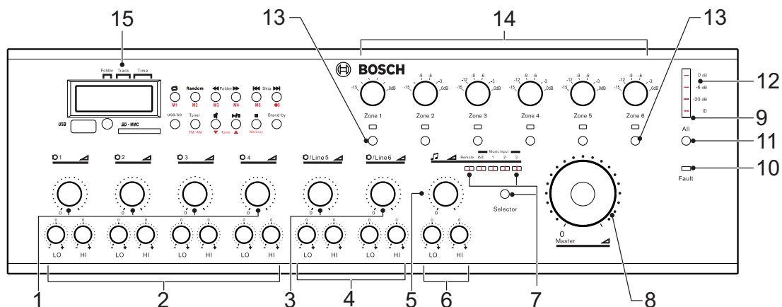
Figura 8.1: Pannello anteriore
