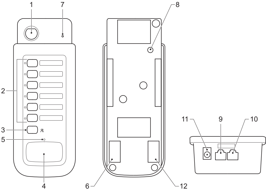
Figura 8.5: Funzioni della stazione di chiamata PLN-6CS
