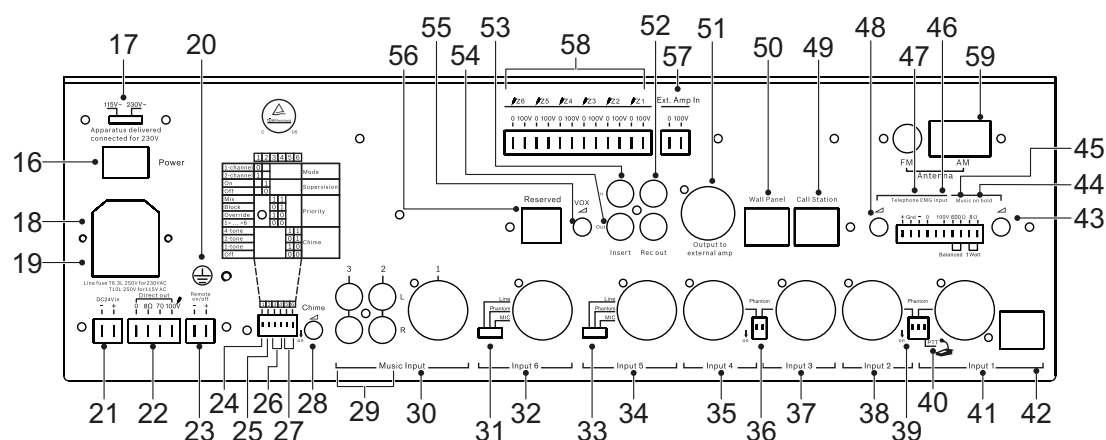
Figura 7.1: Pannello posteriore
