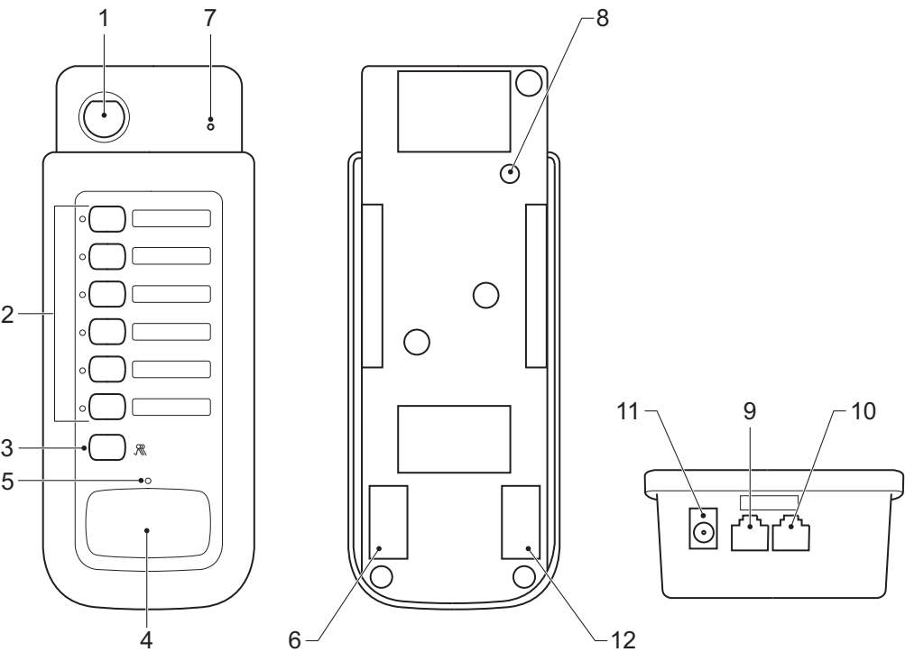
Figura 6.4: Collegamenti della stazione di chiamata PLN-6CS
