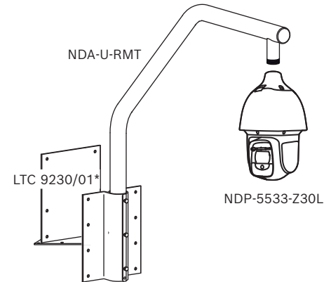
Fig. 3: Montagem em telhados (IP66)
