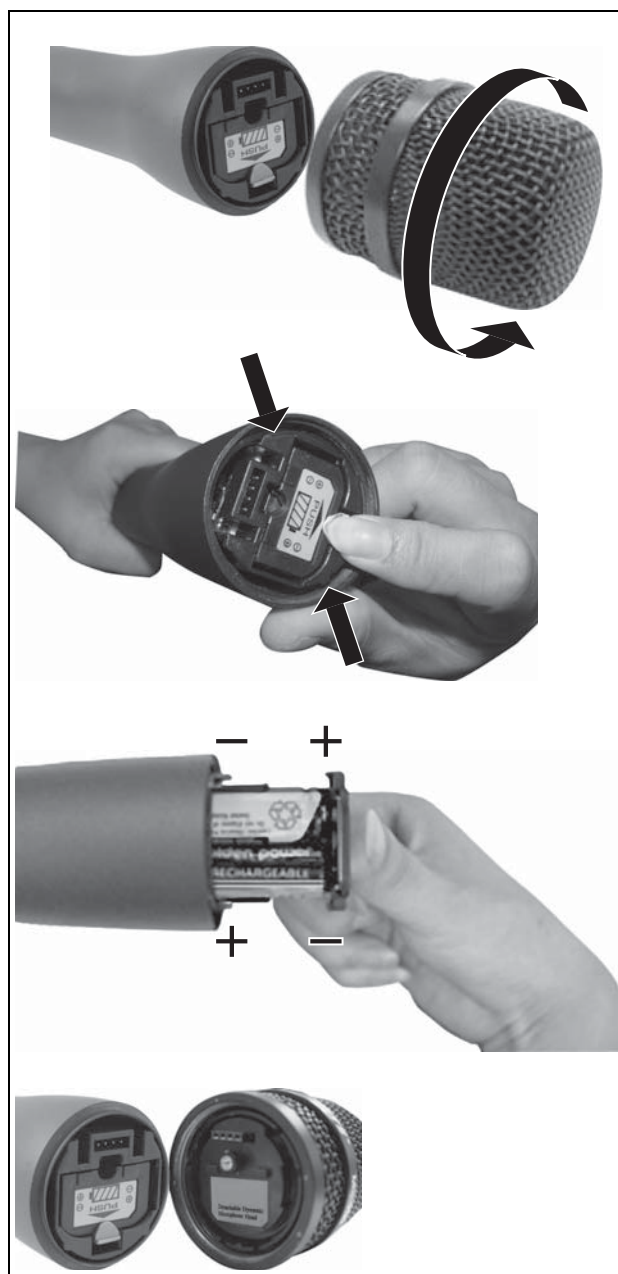
图 4.3: 电池充电 (手持式麦克风)
