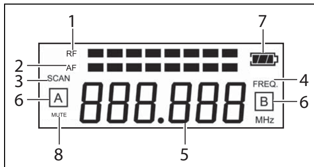
图 3.3: 接收器液晶屏
