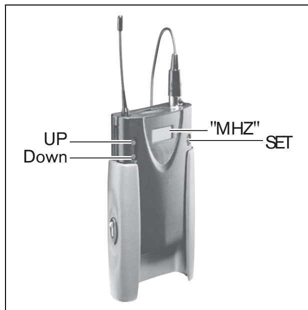
kuva 5.3: Taajuuden säätäminen
