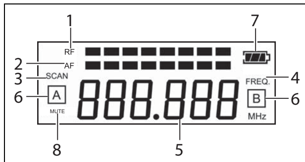
figura 3.3: Ricevitore LCD
