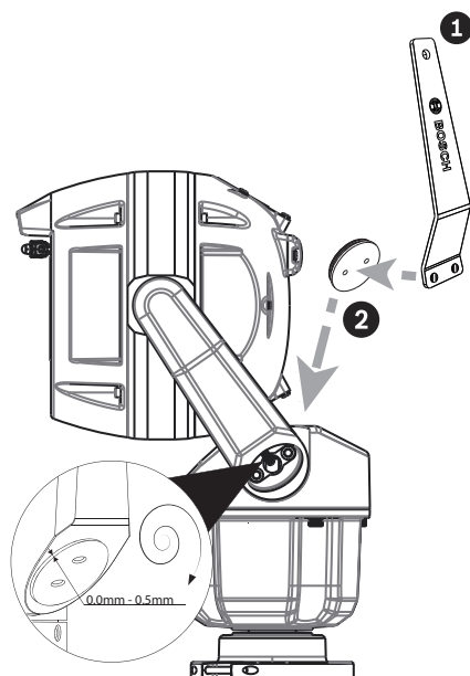
Figura 12.5: Fije las tapas de la horquilla.
