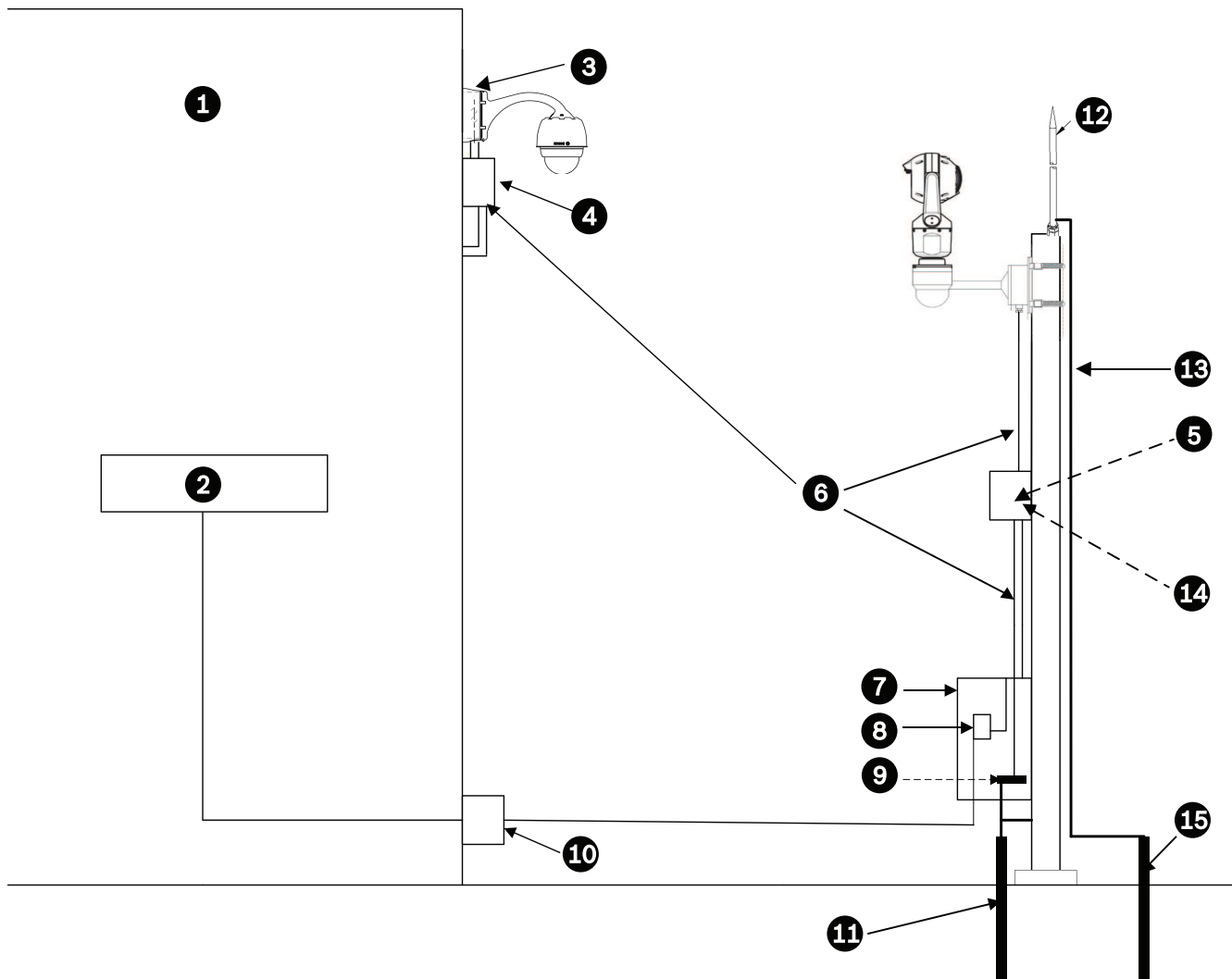
Figur 17.1: Korrekt installation för utomhusbruk med rätt överspännings-/åskskydd
