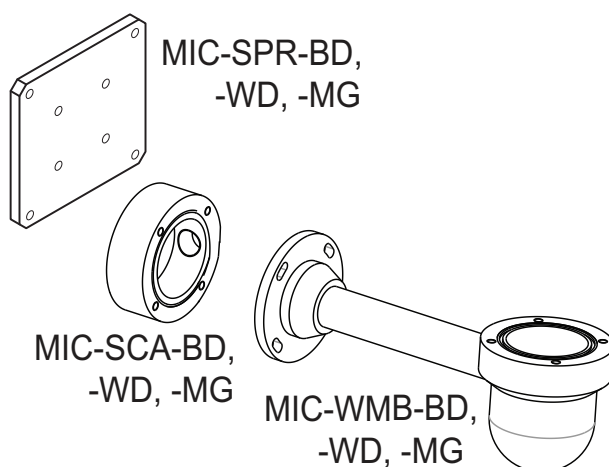
Figur 5.2: Typisk väggmonteringskonfiguration
