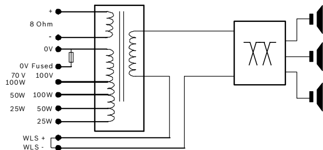
电路图
