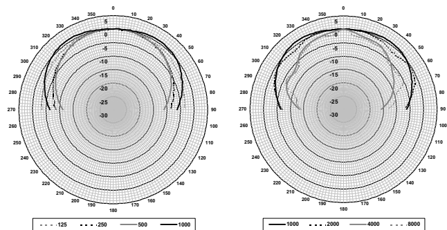
LS1-OC100E-1 的水平指向性图 (粉红噪音, 倍频程, 0° 轴额定值)
