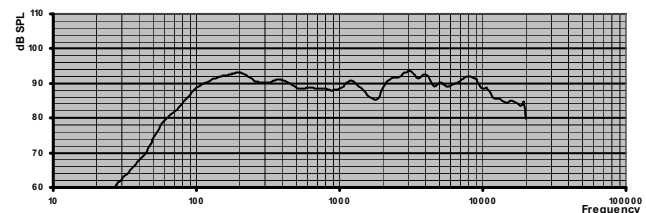
频率响应
