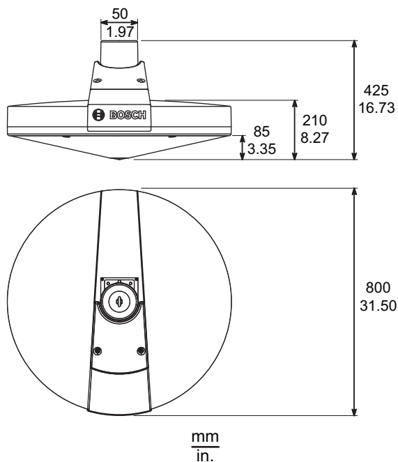
LS1-OC100E-1 尺寸
