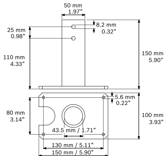
LM1-MSB-1 尺寸
