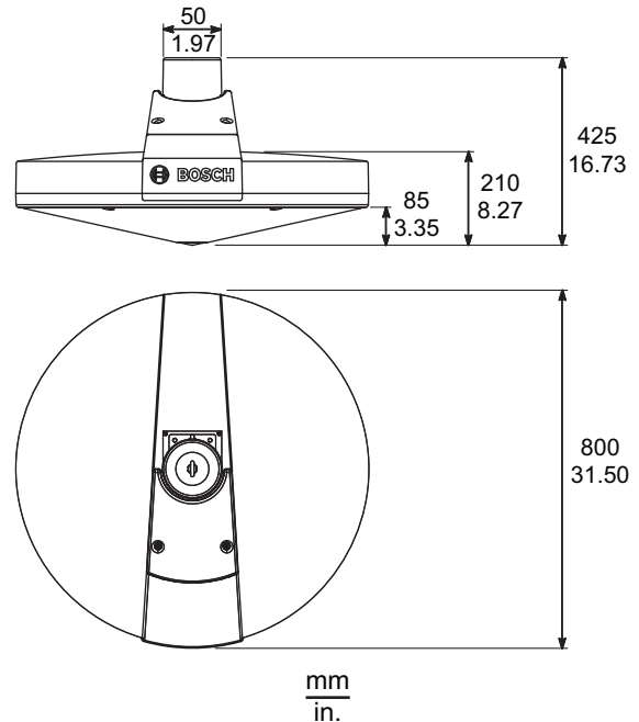
Abmessungen LS1-OC100E-1
