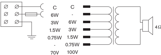
电路图
