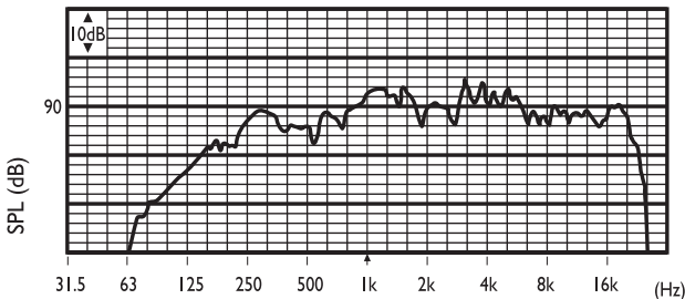
频率响应
