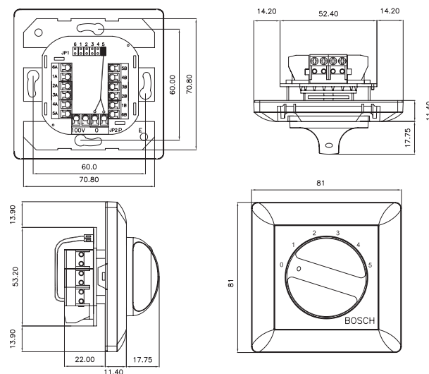
Διαστάσεις του LBC 1431/10 σε mm
