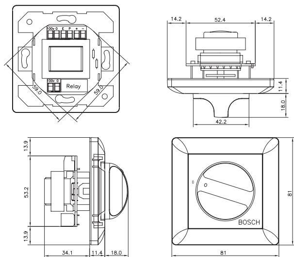
Διαστάσεις των LBC 1411/10 και LBC 1411/20 σε mm
