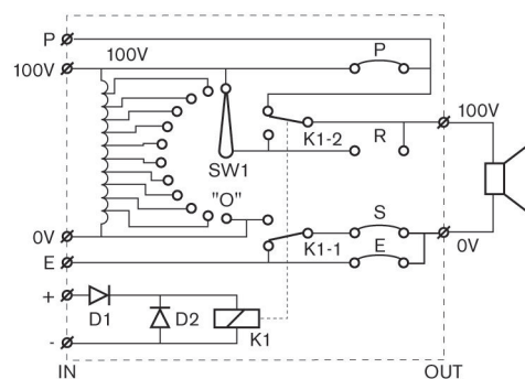
Schéma zapojení LBC 1420/20
