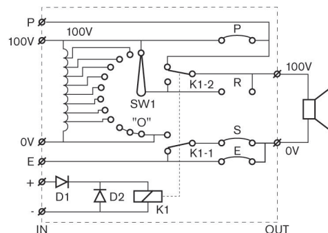
Schéma zapojení LBC 1411/20
