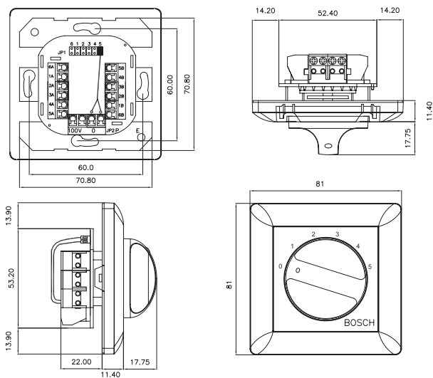
Rozměry LBC 1431/10 v mm
