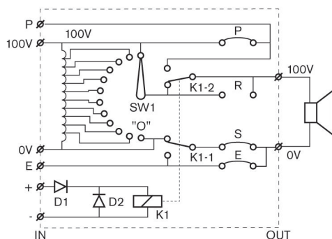
Schéma zapojení LBC 1420/10
