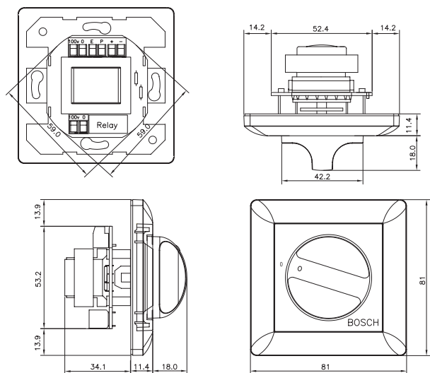
Rozměry LBC 1411/10 a LBC 1411/20 v mm
