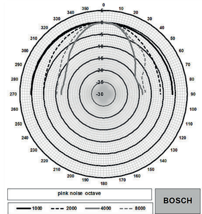
指向性图 (高频部分)
