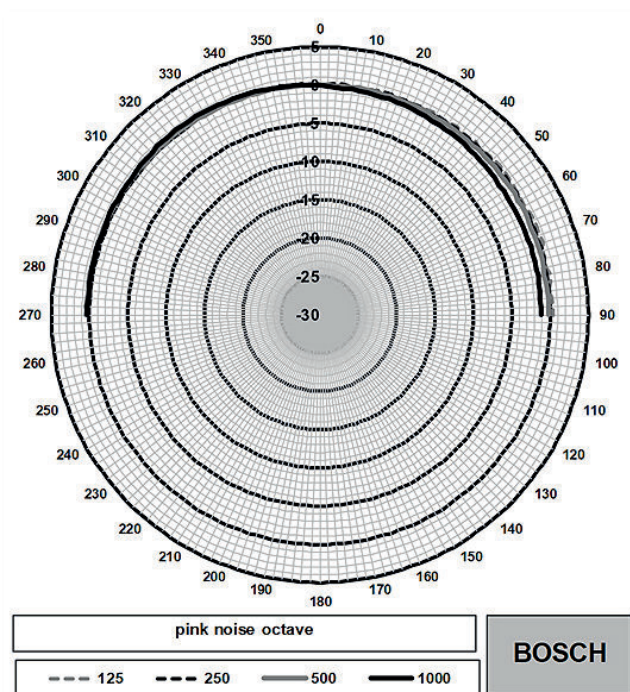
Figura polare (parte bassa frequenza)
