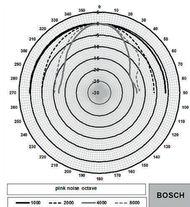
Diagramme polaire (haute fréquence)
