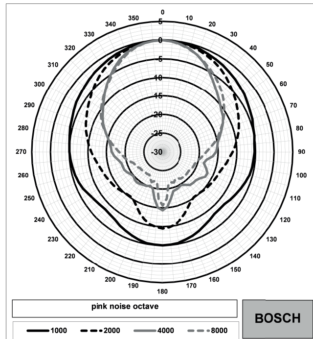
Sơ đồ cực (phần tần số cao)
