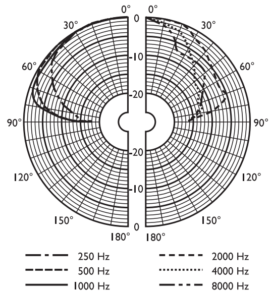
Kuva 5: Suuntakuvi (mitattu vaaleanpunaisella kohinalla)
