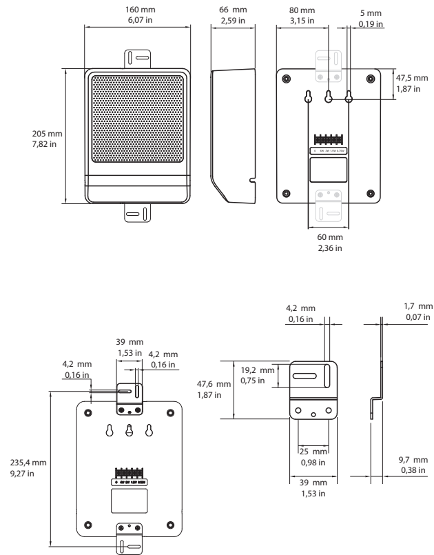
LB10-UC06-Fx dimensions
