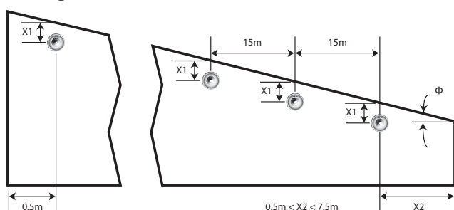
Fig. 5: Montagem em telhado de duas águas
