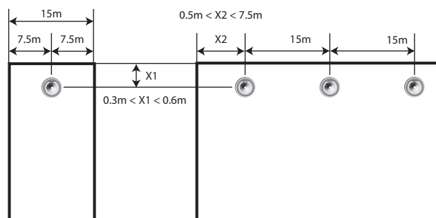
Fig. 3: Montagem em telhado plano
