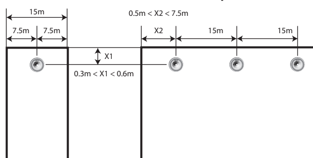
Fig. 3: Montaje en techos planos
