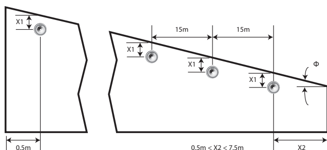
Фиг. 5: Монтаж на двустранно наклонен покрив
