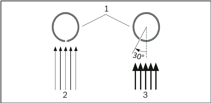
图 5.4 根据气流速度确定空气采样孔的位置
