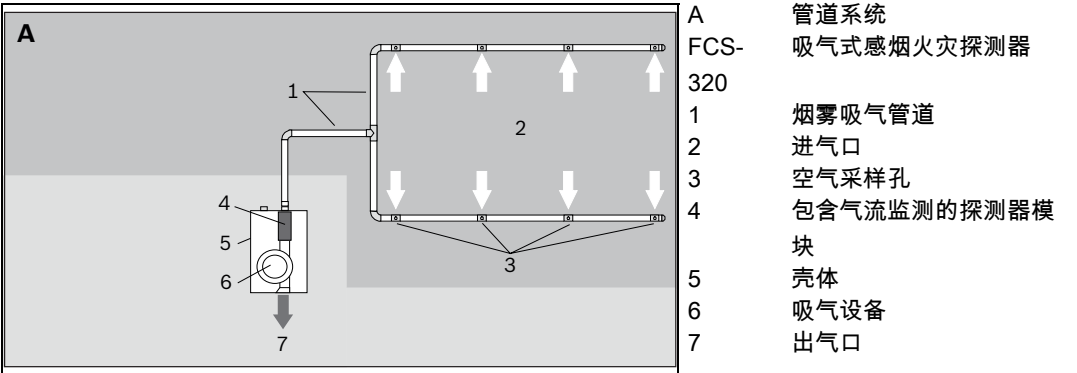
图 2.4 吸气式感烟火灾探测器概述
