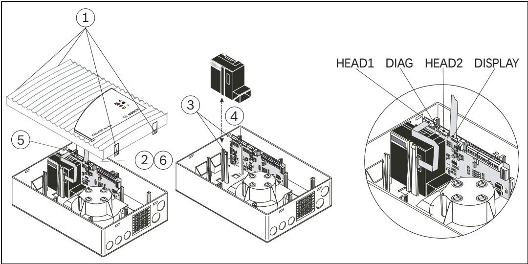
图 4.9 更换探测器模块
