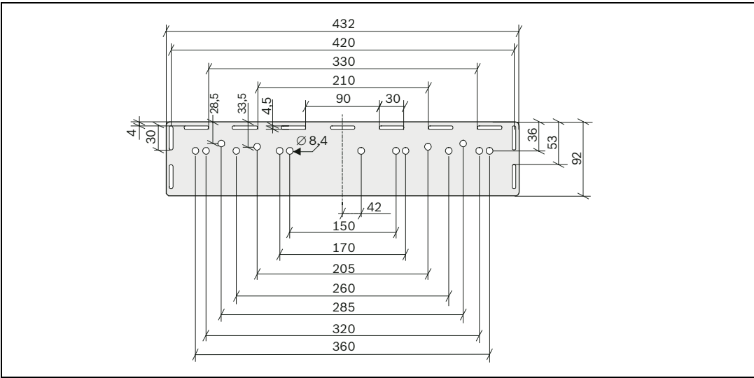
图 4.6 带底座类型 MT-1 的 FCS-320 的孔距
