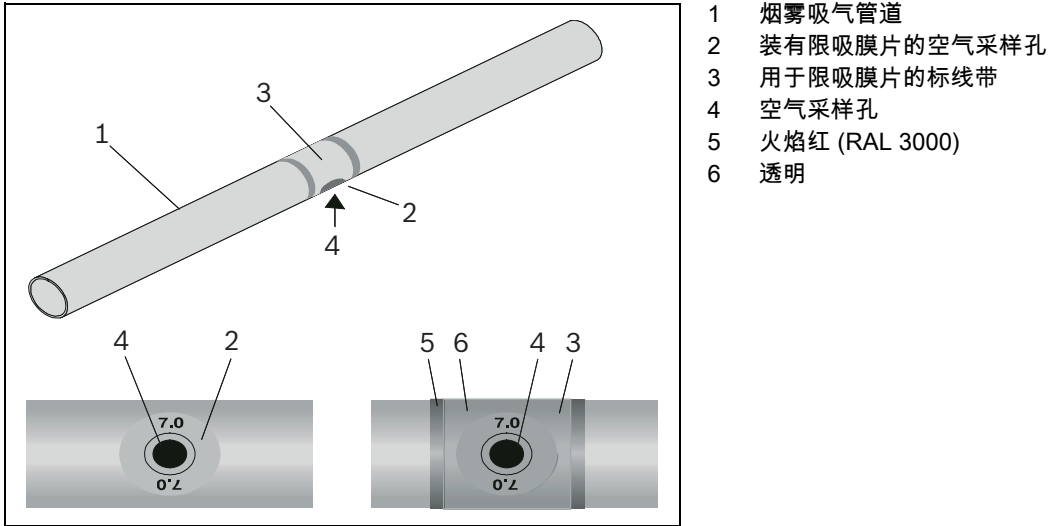
图 2.15 装有限吸膜片和标线带的空气采样孔
