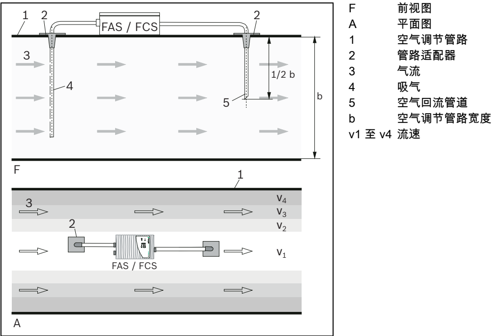
图 3.23 空气回流管道
