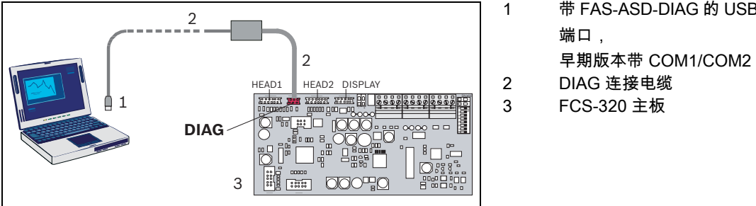
图 4.8 通过诊断电缆连接 PC
