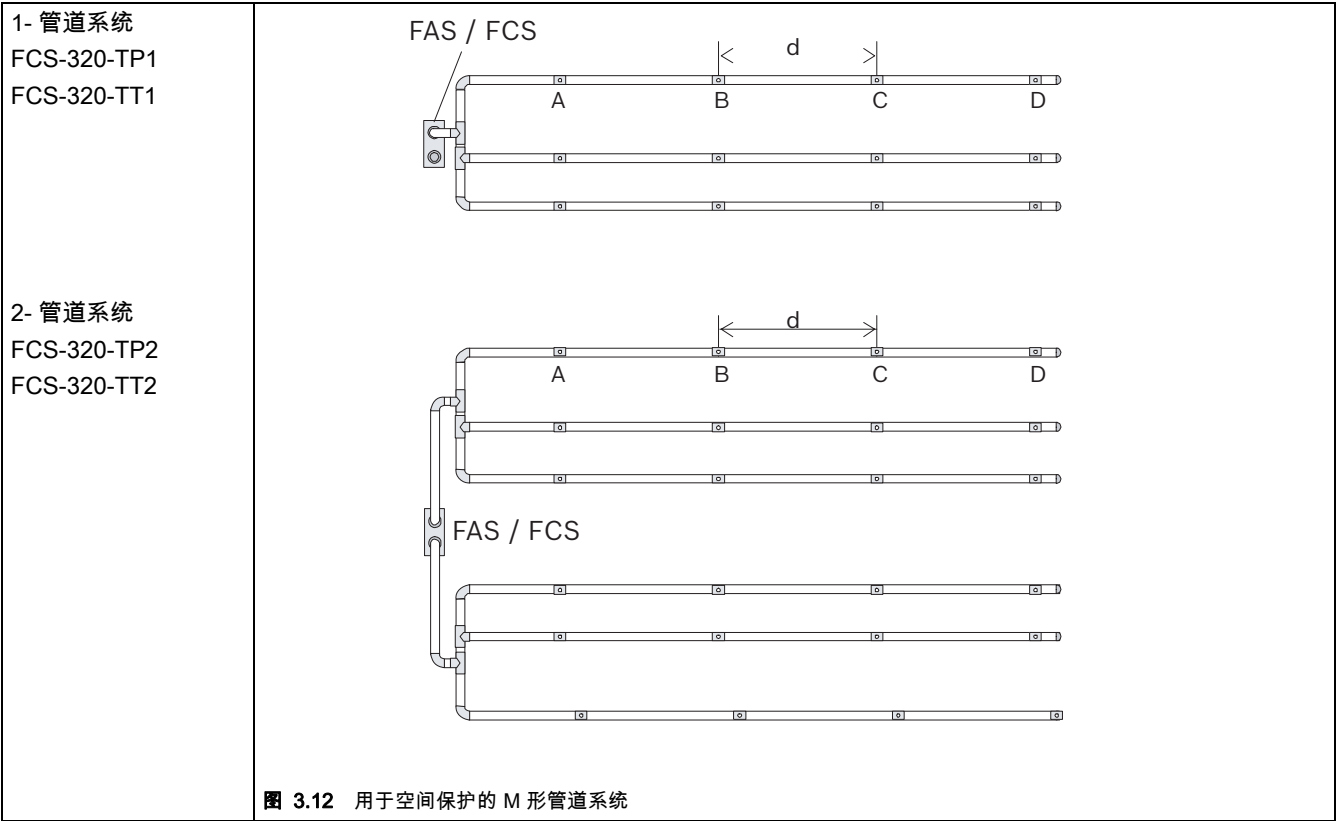
M 形管道系统 - 单孔监测
