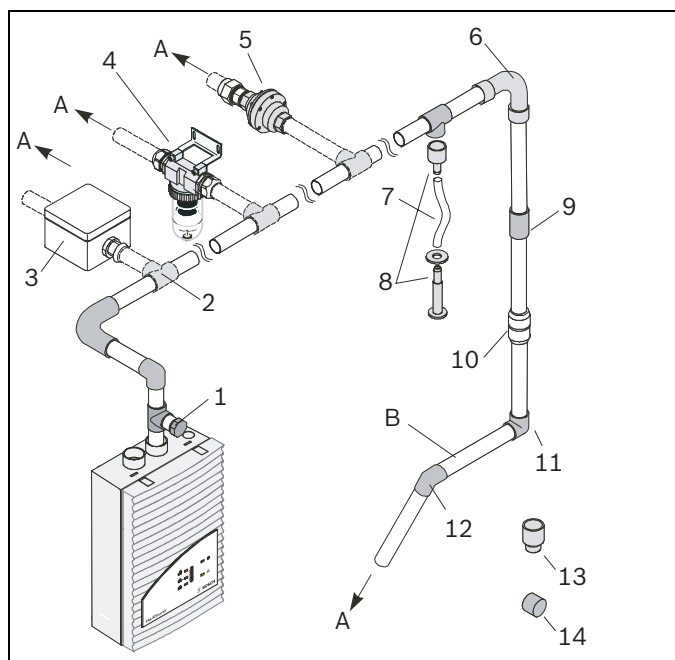
图 2.13 管道系统组件
