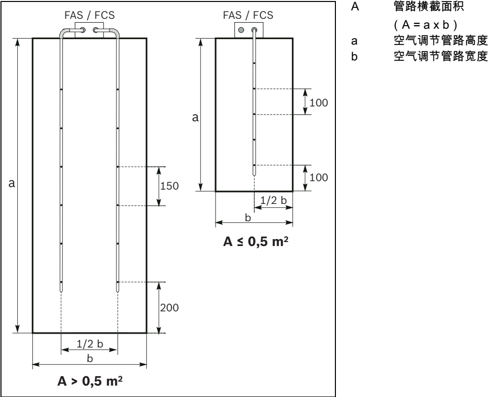
图 3.25 具有小管路横截面和大管路横截面的管路
