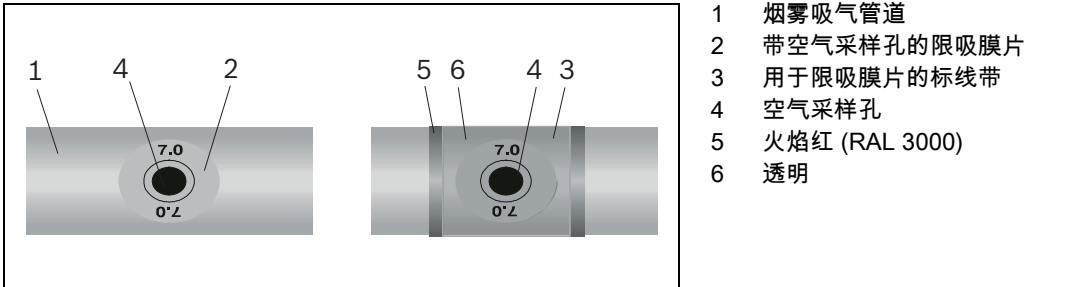
图 5.2 带限吸膜片的吸气孔示例
