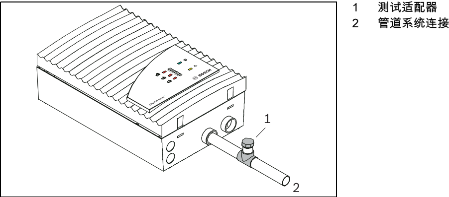
图 5.12 在管道系统中安装测试适配器 要进行测试，只需拔出管道系统连接，并将测试管道直接连接到吸气式感烟火灾探测器。然而，如果吸气管道系统采用永久性安装，则无法进行此测试。此情况下，应使用测试适配器。 测试适配器粘合到管道系统中，紧挨着吸气式感烟火灾探测器。在正常工作中，必须始终关闭测试适配器。仅在维护和保养时才能打开，以便测试气体或烟雾。
