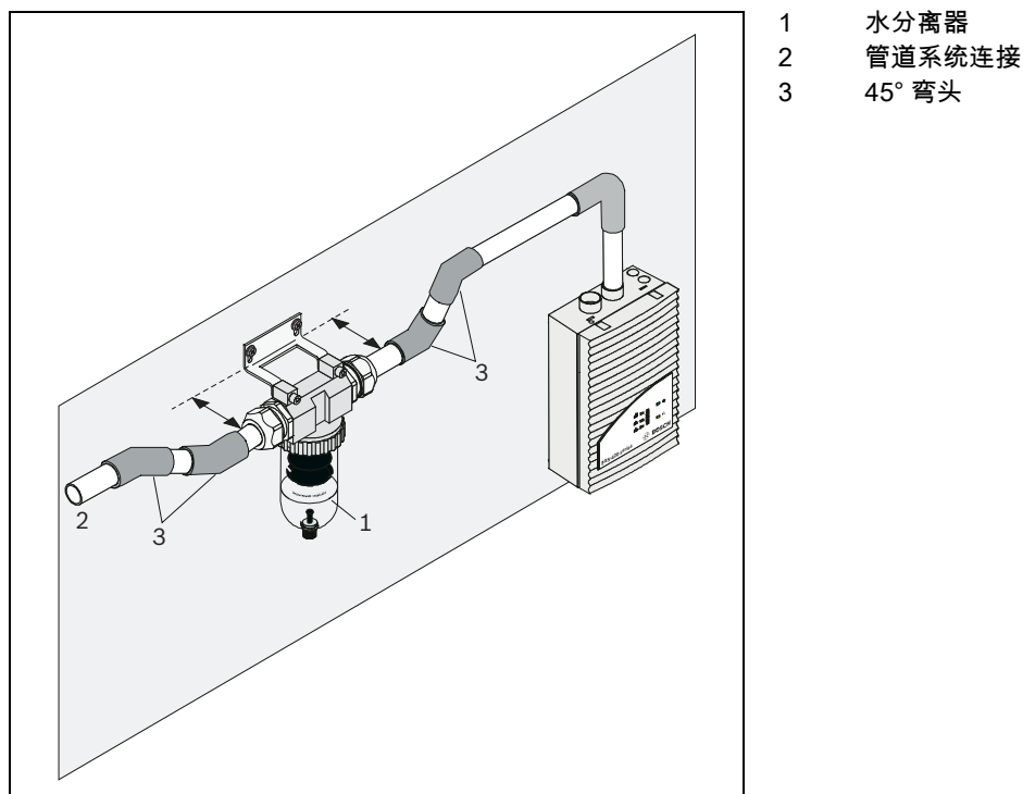
图 2.20 用于蒸发冷凝水并从管道系统收集冷凝水的 FAS-ASD-WS 水分离器
