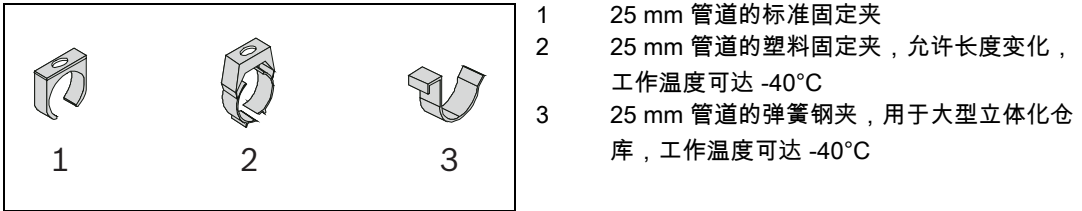
图 5.1 固定夹概览
