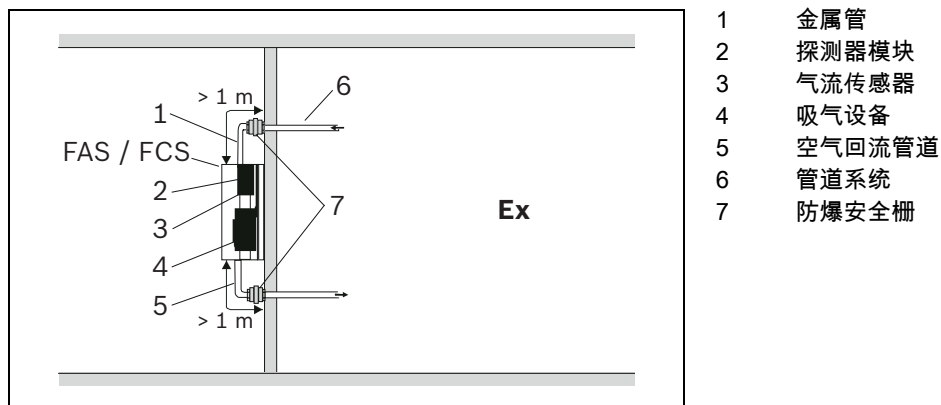
图 2.21 管道系统和（如果需要）空气回流管道中的防爆安全栅
