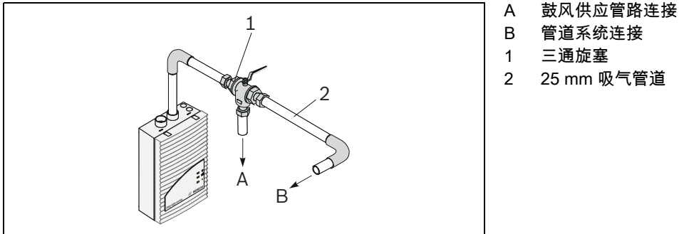
图 2.14 手动吹扫系统组件
