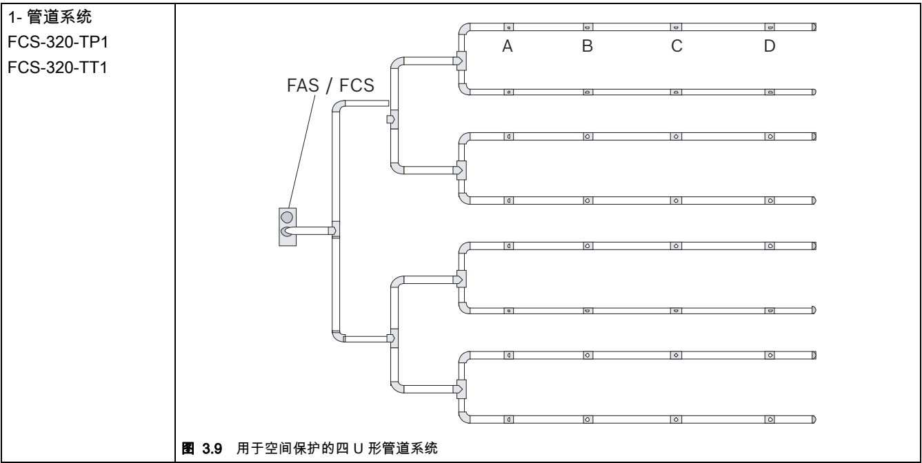
用于空间保护的 四 U 形管道系统
