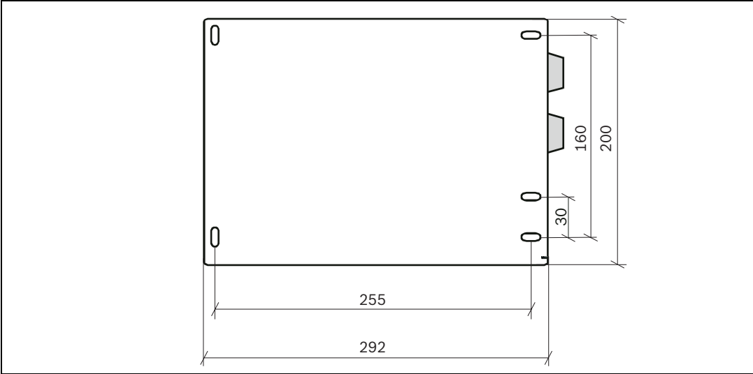
图 4.5 无底座的 FCS-320 的孔距
