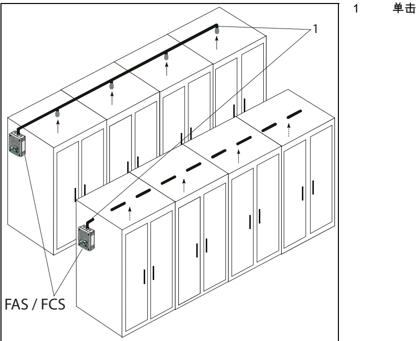
图 2.3 使用 FCS-320 系列吸气式感烟火灾探测器监测设备的原理 FCS-320 系列吸气式感烟火灾探测器还可用于在具有专用空调的区域中进行早期火灾探测。由于具有较高的探测灵敏度，它可以监测高价值的物品和设备。因此 FCS-320 系列特别适合难以探测的应用区域 - 因价值高昂而特别重视早期干预的区域 - 必须确保设备始终正常操作的区域 - 需要较高探测灵敏度的区域（例如，由于内置过滤器设备导致空气中包含的烟雾浓度过低的区域） - 空气交换率较高的区域
