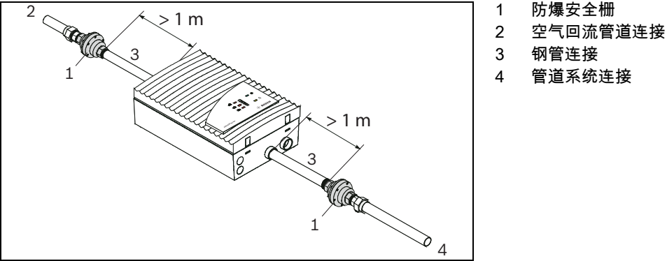
图 5.11 在管道系统和空气回流管道上安装防爆安全栅 防爆安全栅集成在管道系统和空气回流管道中，它与吸气式感烟火灾探测器之间的距离至少 1 m。防爆安全栅通过过渡螺丝连接管连接到管道系统或空气回流管道一侧，并通过钢管连接到 FCS-320 设备（参见图 5.11）。防爆安全栅和钢管 / 过渡螺丝连接管通过 3/4" 螺丝连接管进行连接。
