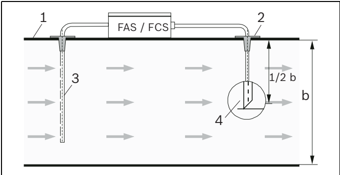
图 5.5 确定空气回流管道的位置 – 空气调节管路（旁路）示例
