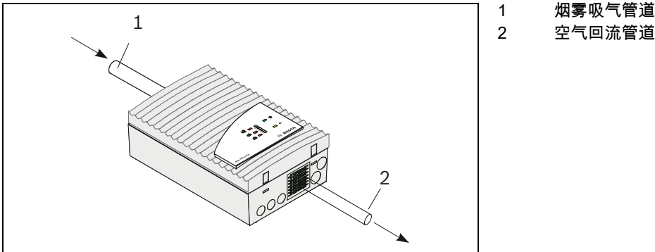
图 2.19 配有空气回流管道的 FCS-320 空气回流管道通过通风格栅连接到 FCS-320 内的排气管（参见图 2.19）。这要求去掉防护格栅中的预冲孔。
