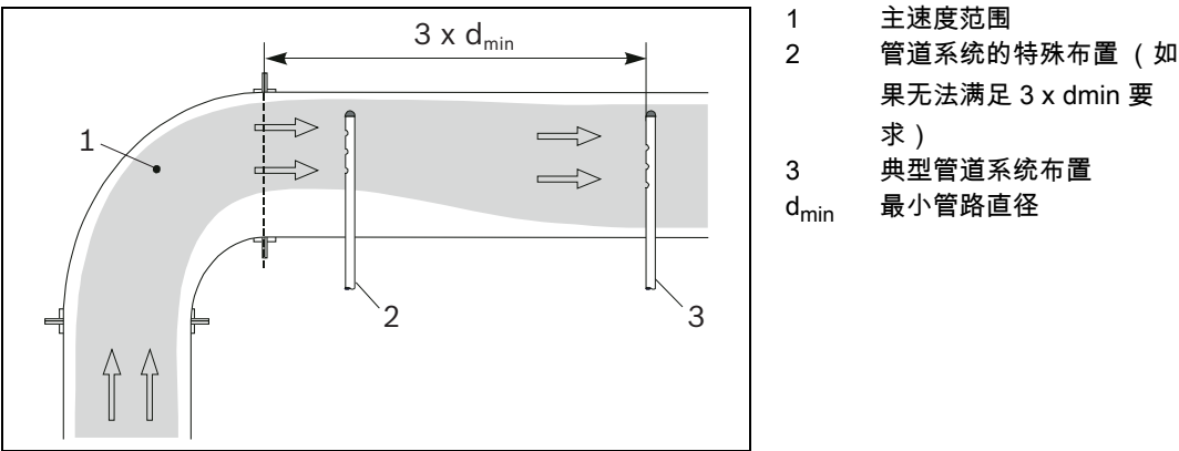
图 3.21 无空气隔板的管路的方向变化
