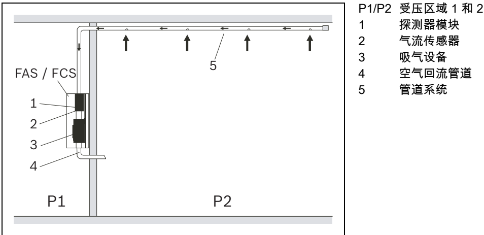
图 2.18 空气回流原理 如果吸气式感烟火灾探测器和管道系统安装在具有不同气压的区域，则吸入的空气必须回流到管道系统的受压区域（参见图 2.18）。空气回流可以平衡气压，或防止邻近空间产生大气负载（例如气味）。
