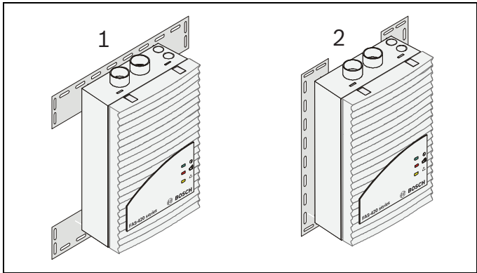
图 4.4 采用底座类型 MT-1 进行安装
