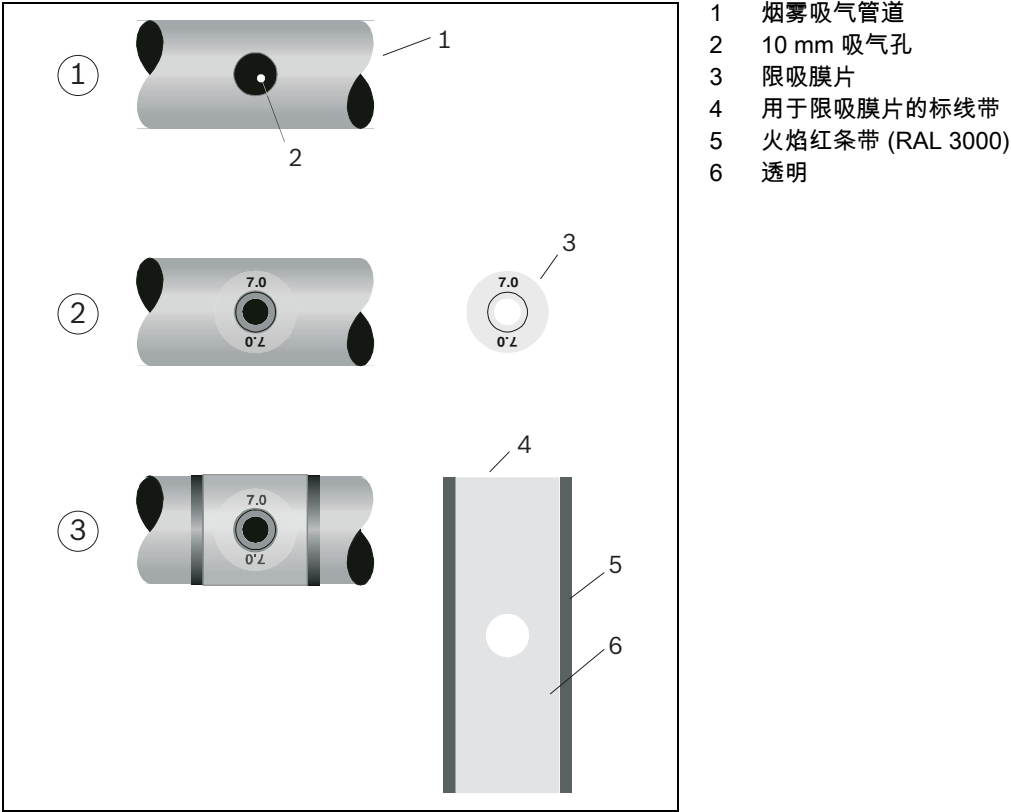
图 5.3 安装限吸膜片
