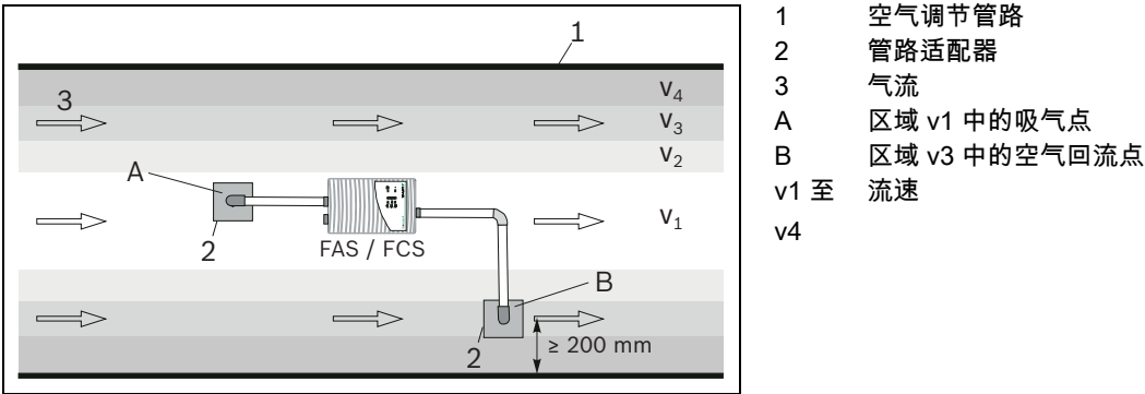
图 3.24 空气回流管道的偏离布置 如果无法满足 2 m 的距离要求，则必须以偏离方式布置管道。这样，由于管道位于不同的速度区域，可以实现进气点和排气点之间的压差（参见图 3.24）。 下表列出了空气采样孔之间的距离以及空气采样孔与管路壁之间的距离。
