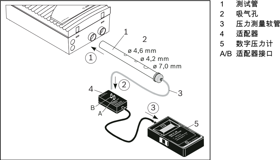
图 6.3 测试 FCS-320 的可操作性
