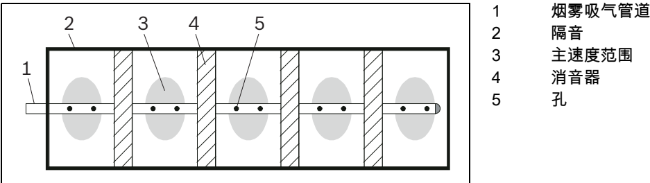
图 3.22 管路中的消音器
