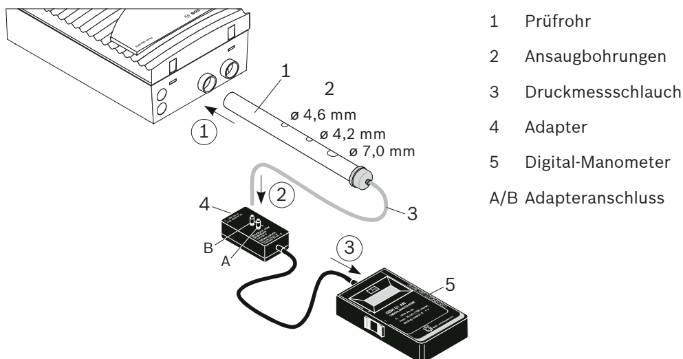
Prüfen der Funktionsfähigkeit des FCS-320
