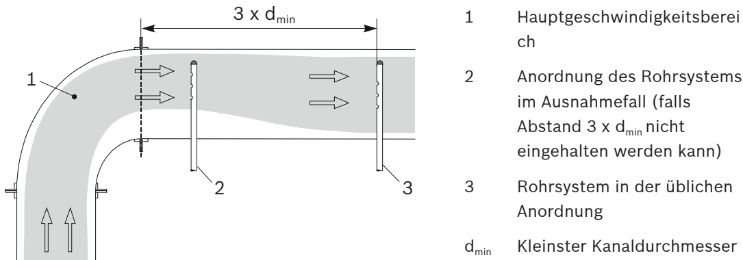
Richtungsänderung des Kanals ohne Leitbleche
