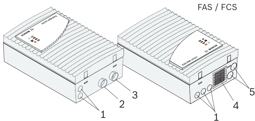
Abbildung 3.1: FCS-320 Anschlüsse
