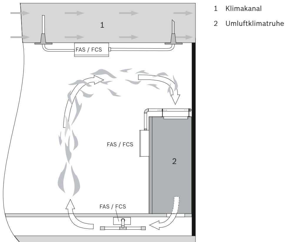
Überwachungsmöglichkeiten einer Klimatrube bzw. eines Klimakanals (Prinzipdarstellung)
