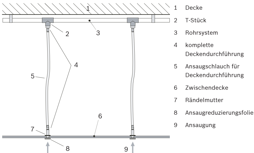
Deckendurchführungen
