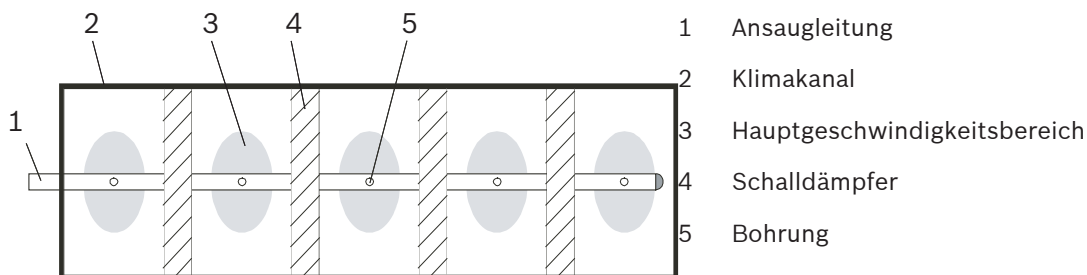
Schalldämpfer in einem Kanal
