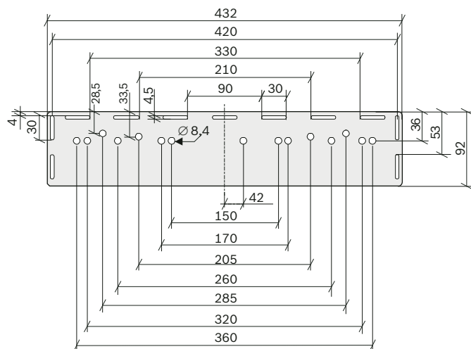
Abbildung 5.2: Bohrabstände der Halterung Typ MT-1
