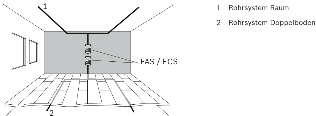
Prinzip der Raumüberwachung mit Ansaugrauchmeldern der Serie FCS-320
