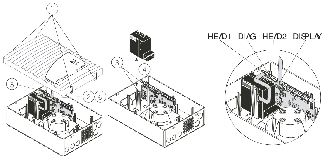
Austausch eines Detektormoduls
