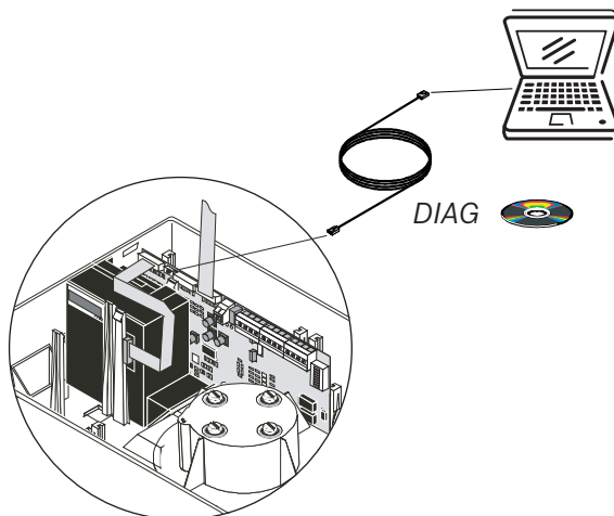
Abbildung 3.4: Diagnosesoftware zum Auslesen des Gerätezustands
