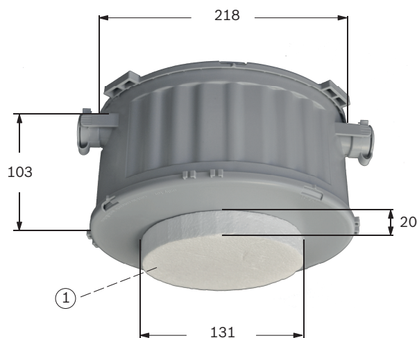
Figura 3.10: Alloggiamento integrato FAA-500-CB
