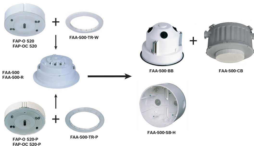
Figura 1.2: Rivelatori ed accessori serie 520
