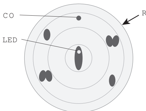
Figura 5.1: Posizione dell'interruttore reed
