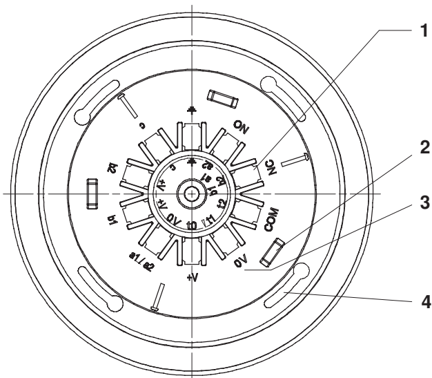
Figura 3.5: Vista dall'alto della base
