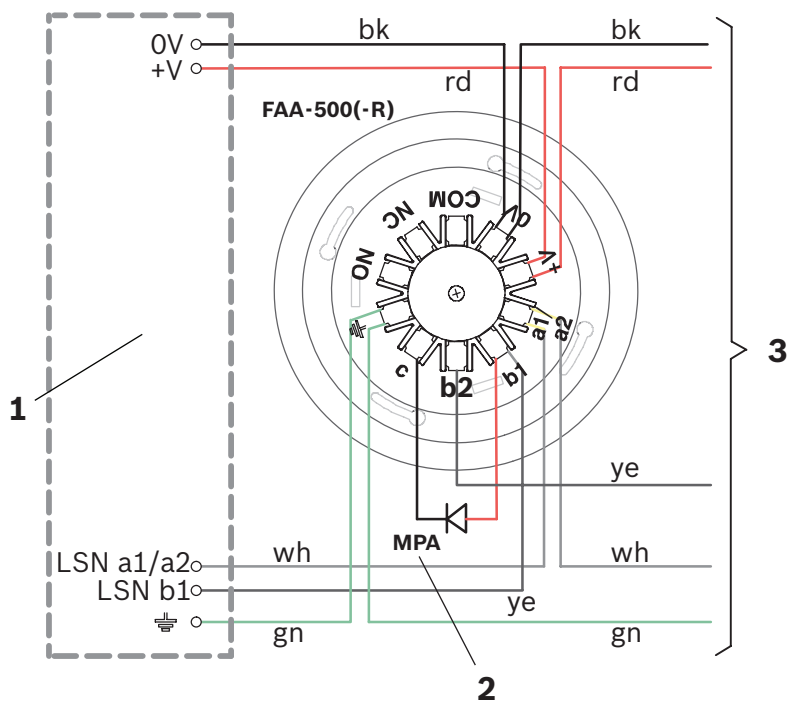
Figura 3.6: Collegamento delle basi
