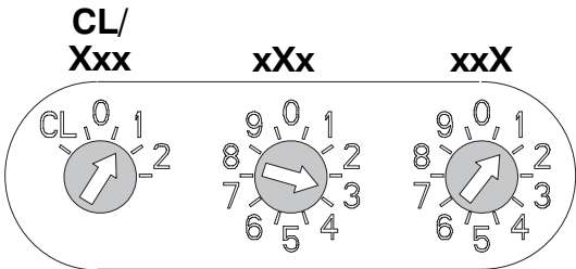
Figura 3.8: Interruttore a rotazione
