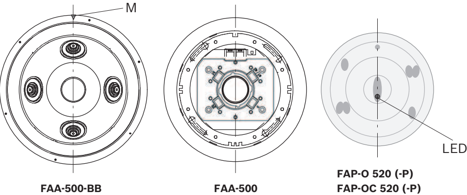
Figura 3.3: Allineamento della scatola posteriore per montaggio a soffitto, base e rivelatore
