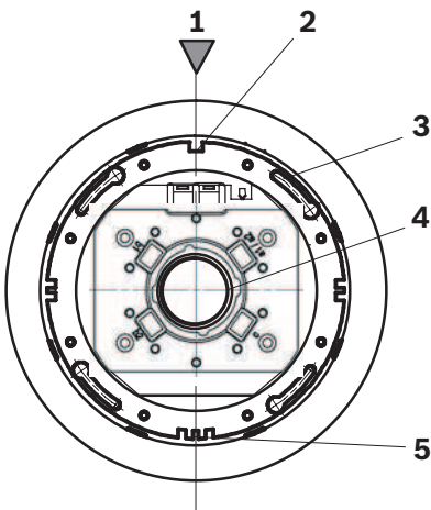
Figura 3.7: Posizionamento della base nella scatola posteriore per montaggio a soffitto
