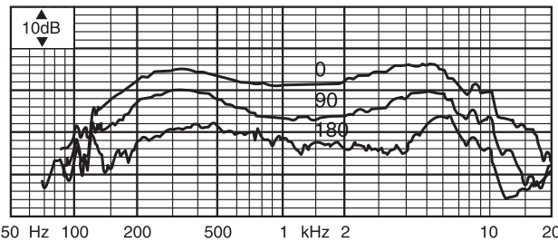
频率响应
