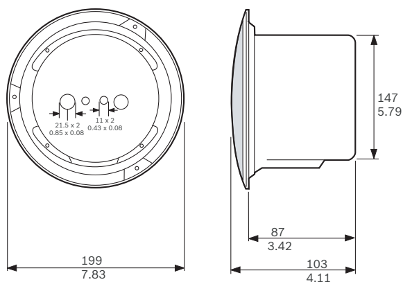
Kích thước của bộ vòm chống cháy LHM 0626/00 và LBC 3080/01 tính theo mm (in)
