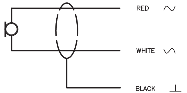
Devre şeması
