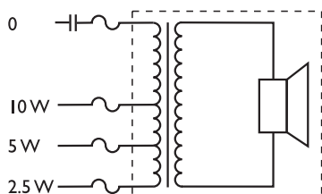
Принципиальная схема
