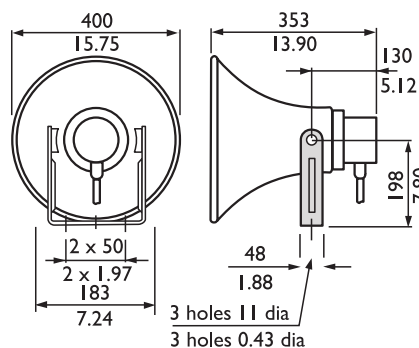
Размеры (мм)
