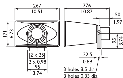
Размеры (мм)
