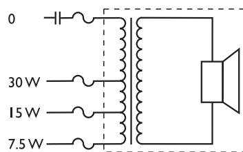
Принципиальная схема
