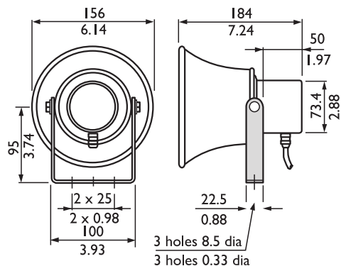
Размеры (мм)
