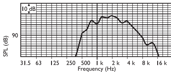
Частотная характеристика
