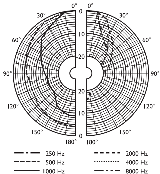
Горизонтальная полярная диаграмма (для розового шума)
