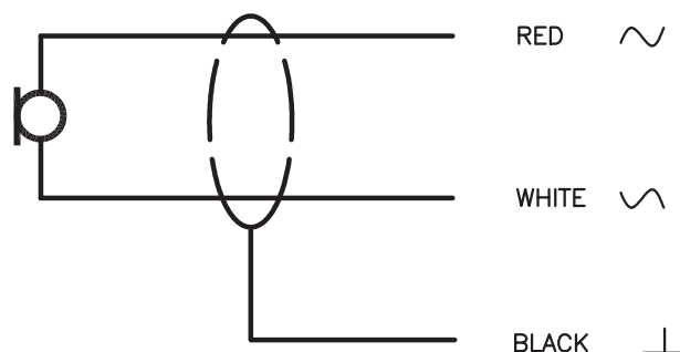
Diagramme électrique
