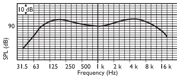
Taajuusvaste
