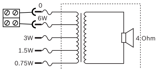
KytKentäkaavio
