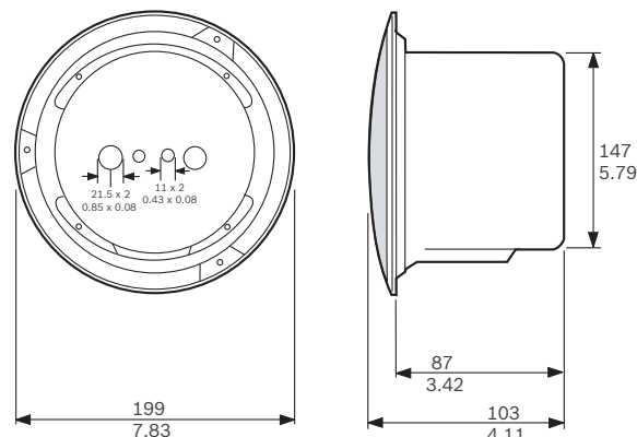
LHM-0626/00 + LBC 3080/01 -palokupu, mitat
