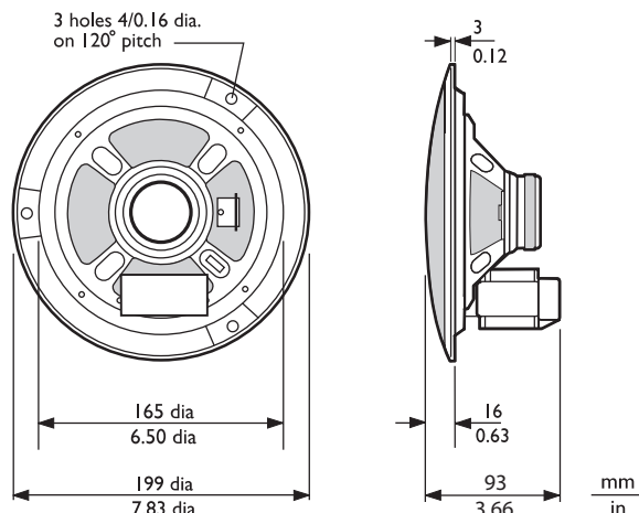
Mitat millimetreinä
