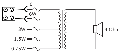
Schéma zapojení
