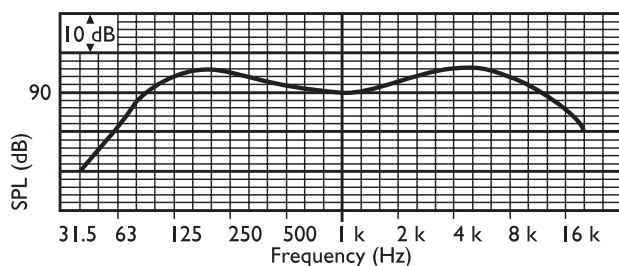
Kmitočtová charakteristika
