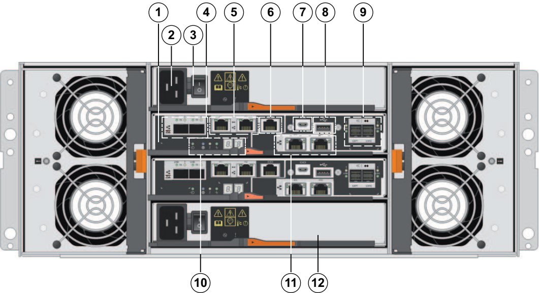
Unidade de controlador duplo de 60 compartimentos - visão traseira
