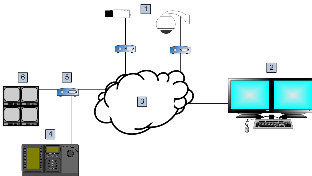
Рис. 5.2: Сценарий 2: клавиатура Bosch IntuiKey, подключенная к декодеру
