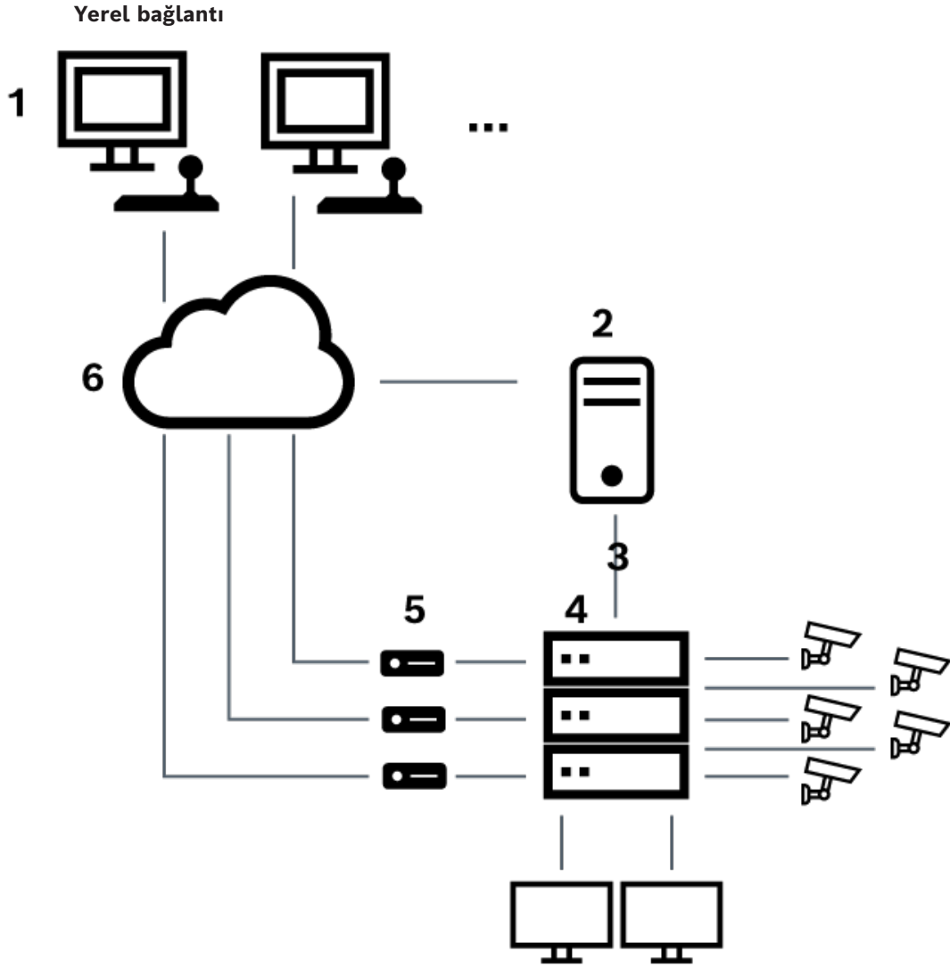
Şekil 6.3: Bosch Video Management System'in Bosch Allegiant matris anahtarına yerel bağlantısı
