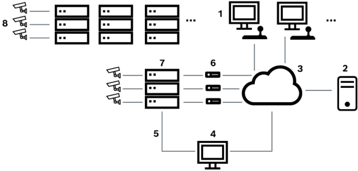
Şekil 6.5: Satellite anahtarlarıyla genişletilmiş Bosch Allegiant sistemi
