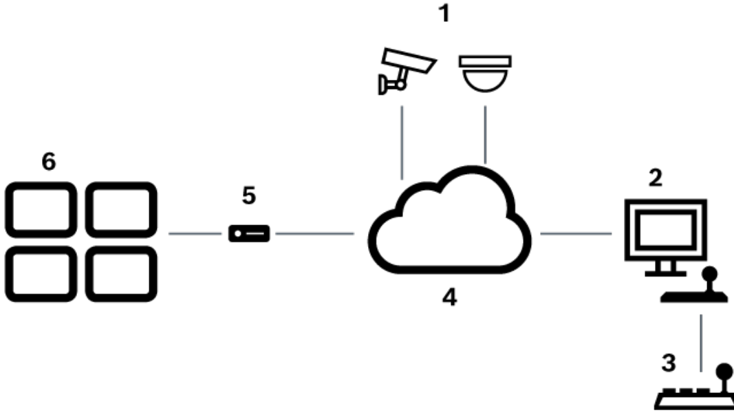
Şekil 6.1: 1. Senaryo: Bosch Video Management System iş istasyonuna bağlı Bosch IntuiKey klavye
