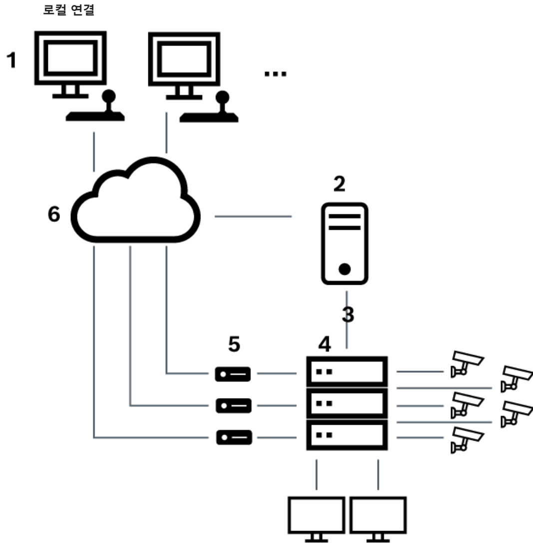
그림 6.3: Bosch Allegiant 매트릭스 스위치에 대한 Bosch Video Management System 로컬 연결
