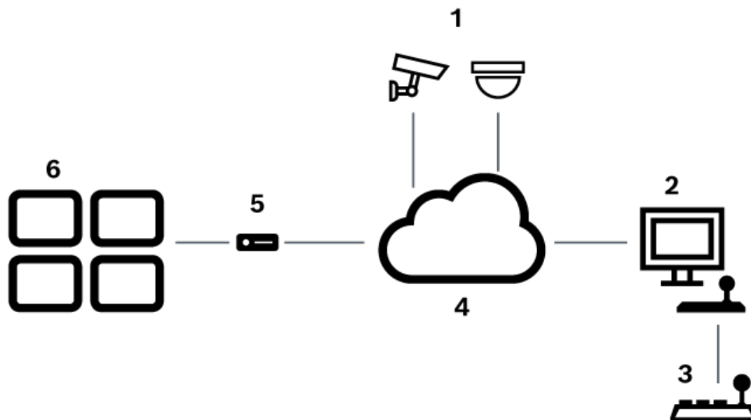
그림 6.1: 시나리오 1: Bosch Video Management System 워크스테이션에 연결된 Bosch IntuiKey 키보드
