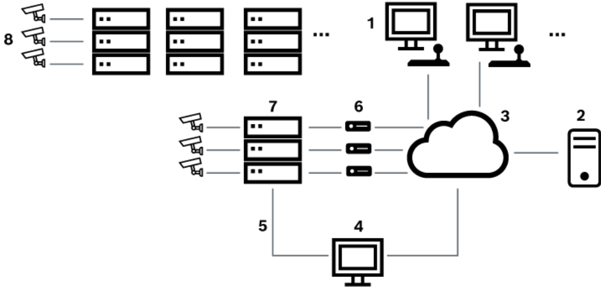
그림 6.5: 위성 스위치로 확장된 Bosch Allegiant 시스템
