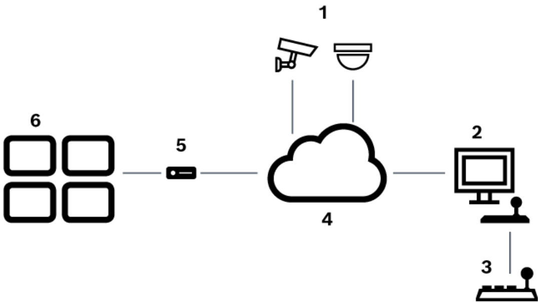
Abbildung 5.1: Szenario 1: An eine Bosch Video Management System Arbeitsstation angeschlossenes Bosch IntuiKey Keyboard
