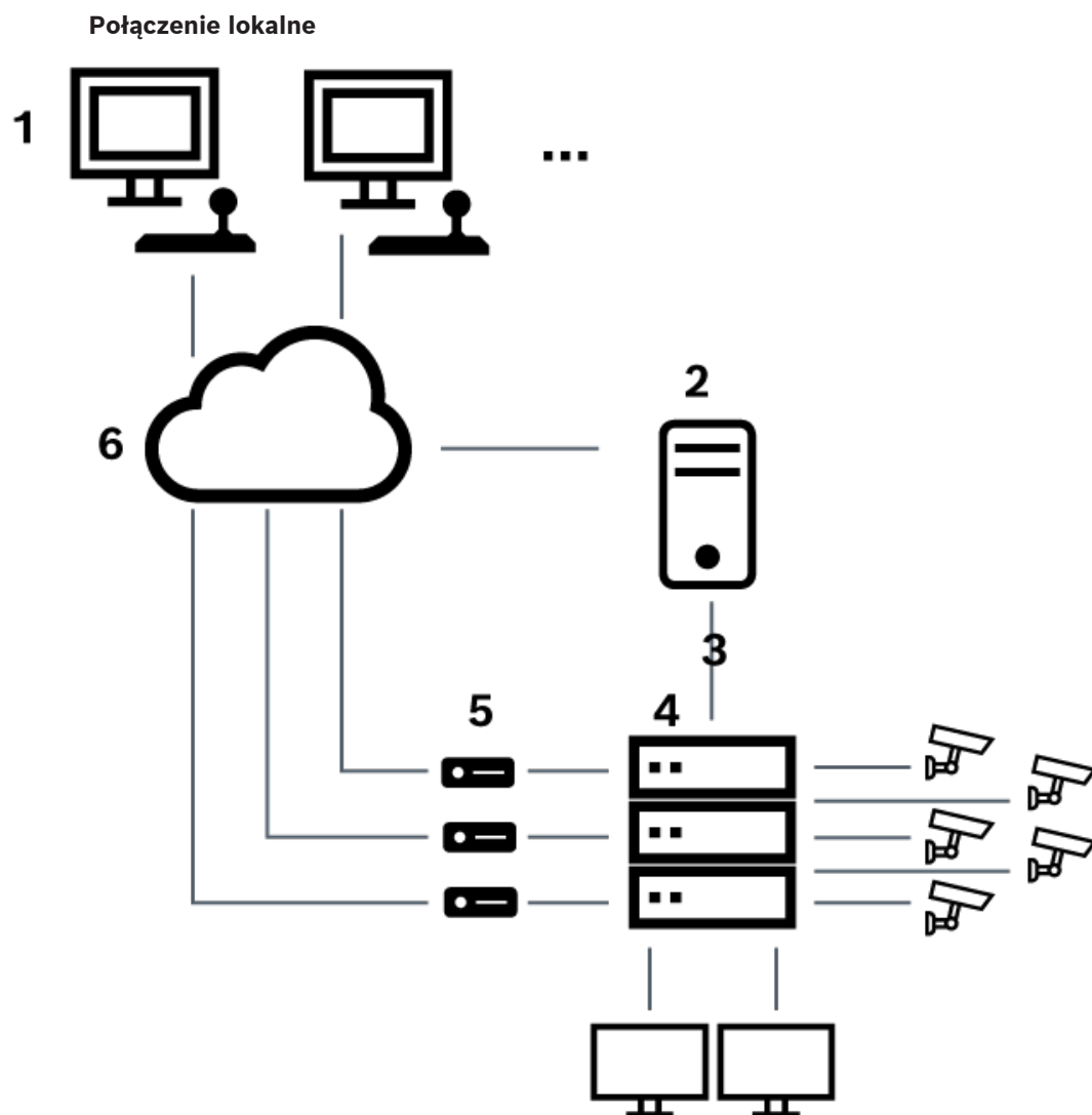
Rysunek 5.3: Lokalne połączenie systemu BVMS z krosownicą Bosch Allegiant
