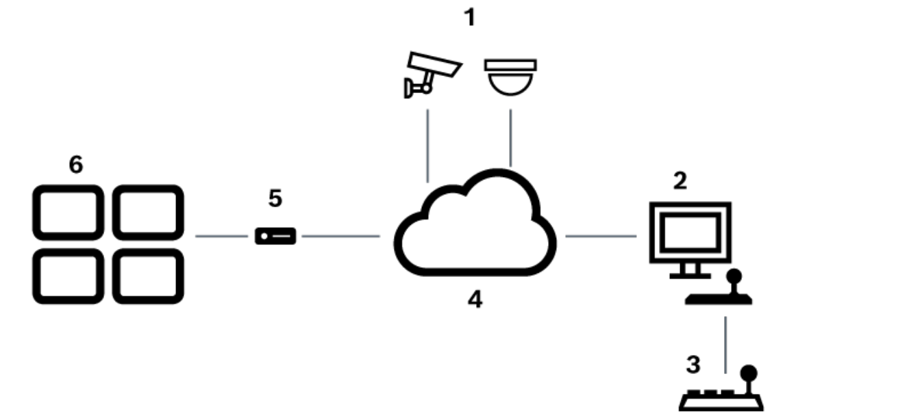
Figura 5.1: Escenario 1: teclado IntuiKey de Bosch conectado a una estación de trabajo de Bosch Video Management System
