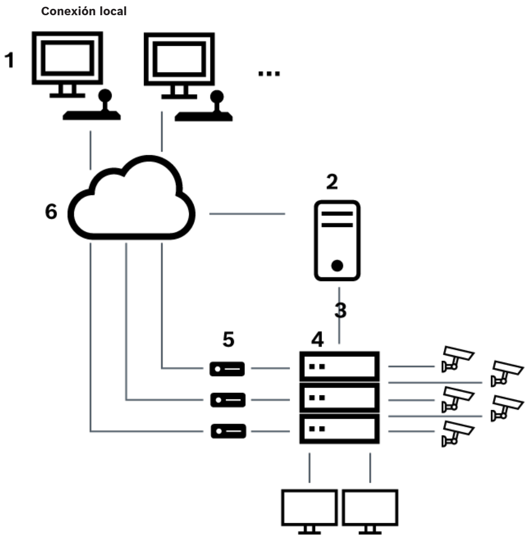
Figura 5.3: Conexión local de Bosch Video Management System a una matriz Allegiant de Bosch
