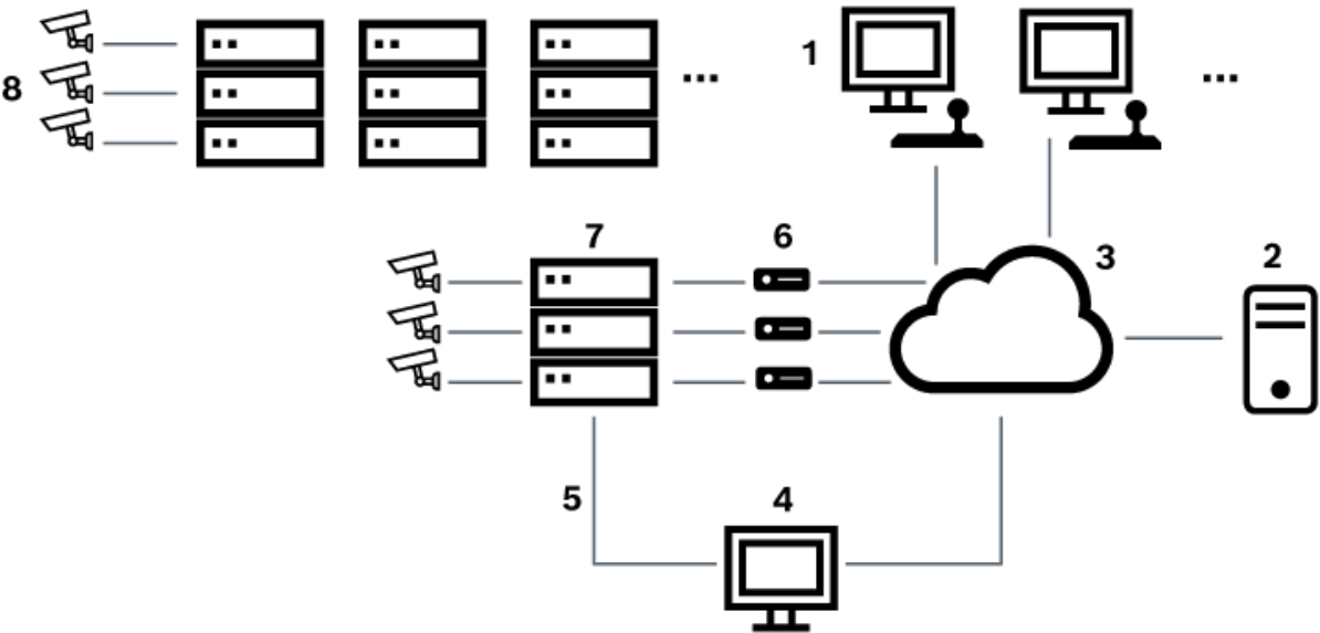
Figura 5.5: Sistema Bosch Allegiant ampliado con matrices satélite
