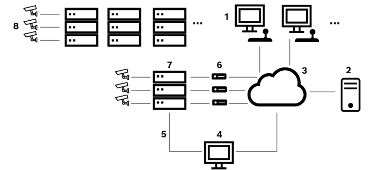
Attēls 5.5: Bosch Allegiant sistēma, kas paplašināta ar satelīta slēdžiem
