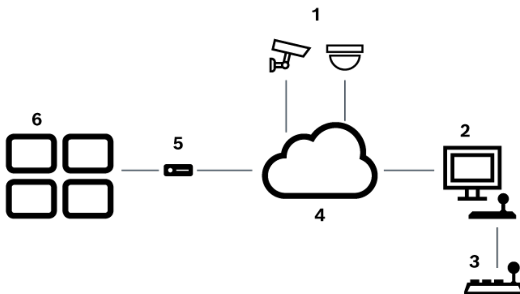
Attēls 5.1: 1. scenārijs: Bosch IntuiKey tastatūra, kas savienota ar Bosch Video Management System darbstaciju
