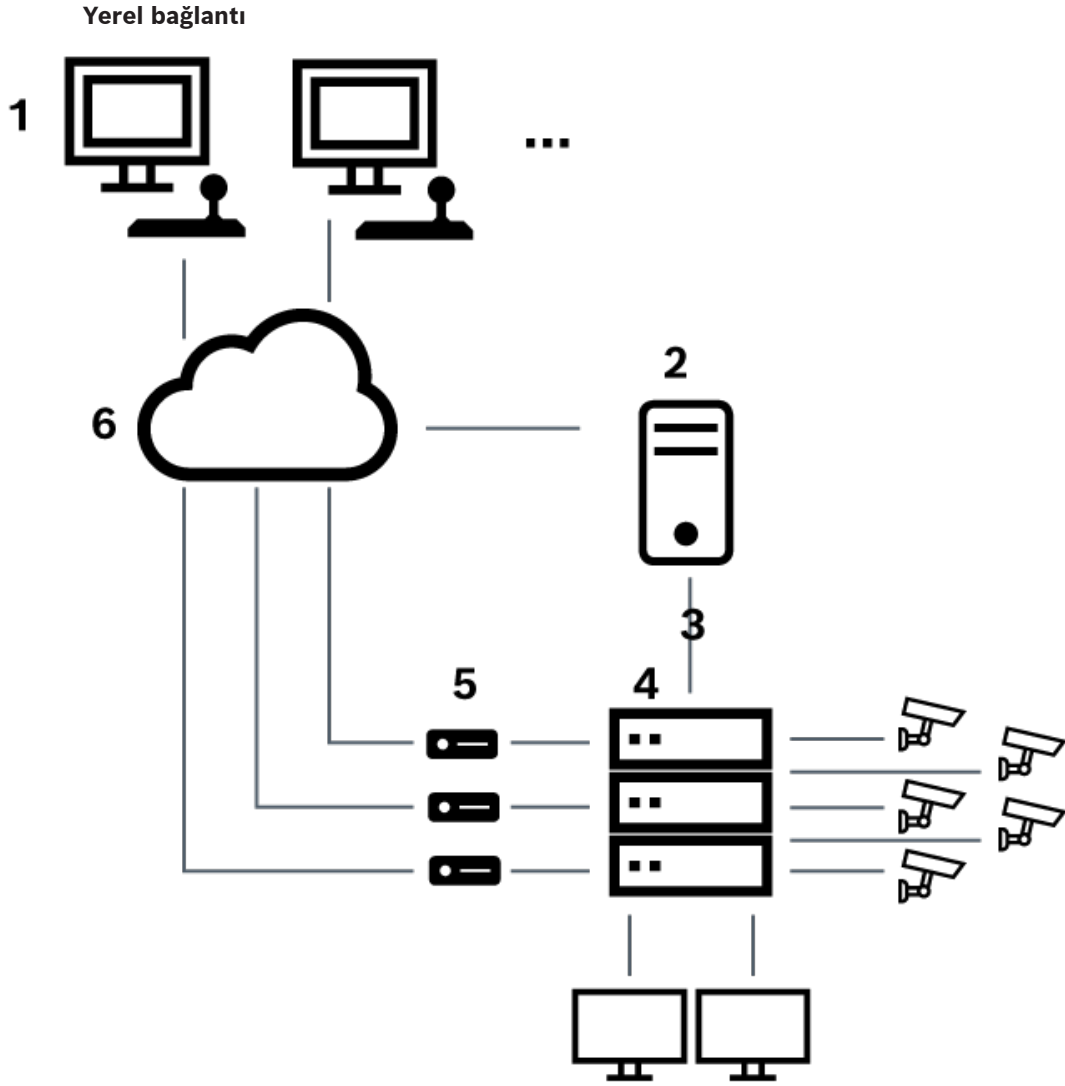
Şekil 5.3: Bosch Video Managem System'in Bosch Allegiant matris anahtarına yerel bağlantısı
