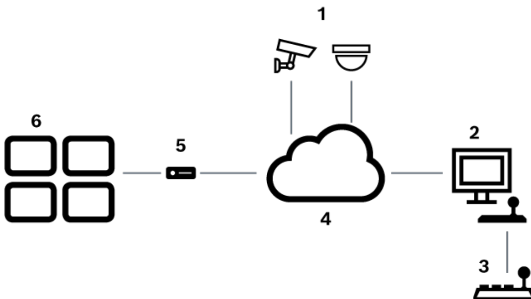
Figura 5.1: Scenario 1: tastiera Bosch IntuiKey collegata a una workstation Bosch Video Management System
