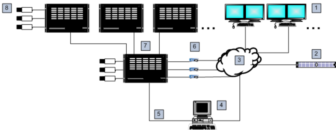
Afbeelding 5.5: Bosch Allegiant-systeem uitgebreid met satellietenschakelaars
