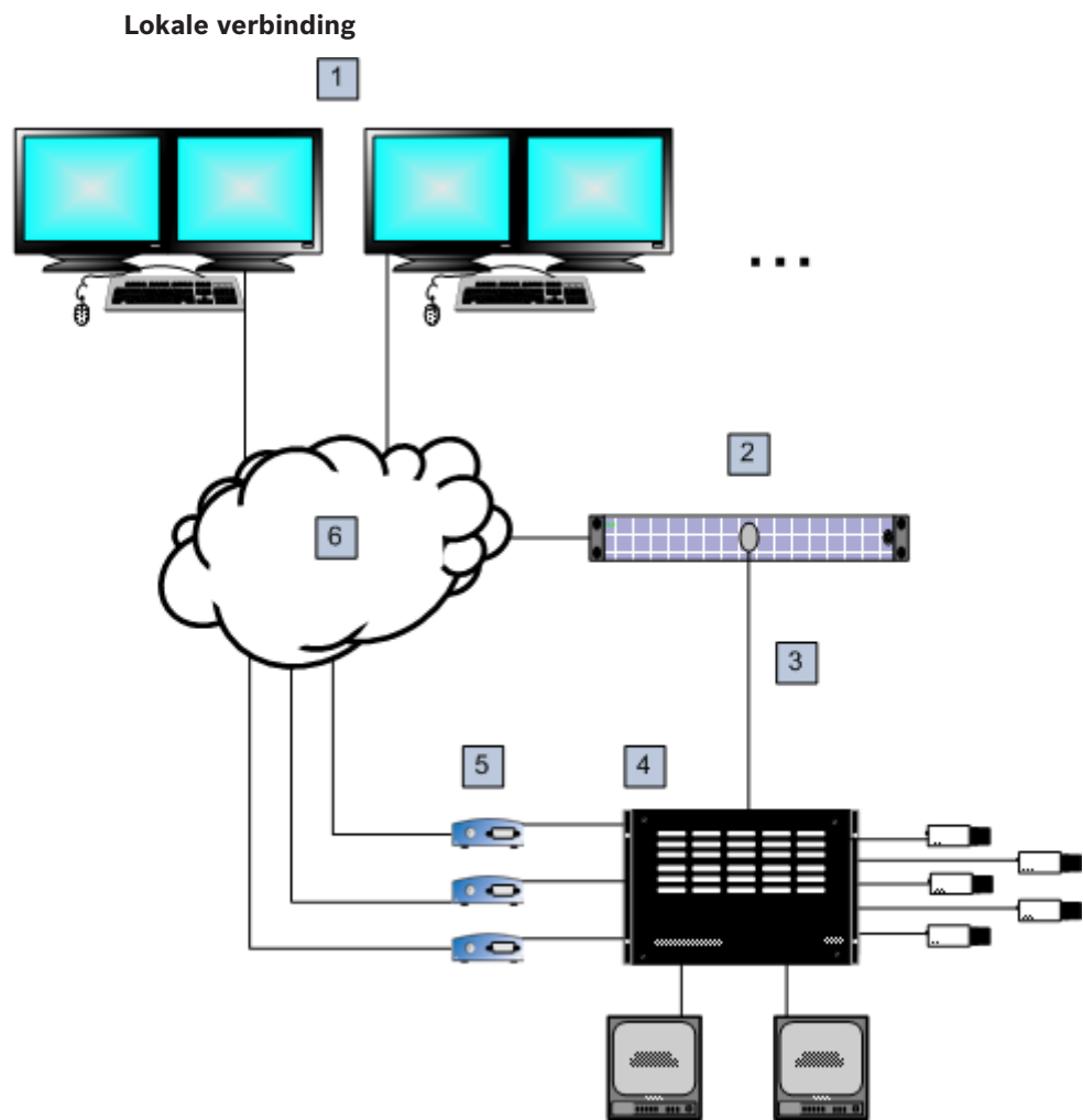
Afbeelding 5.3: Lokale verbinding van een Bosch Video Management System met een Bosch Allegiant Matrix-schakelaar
