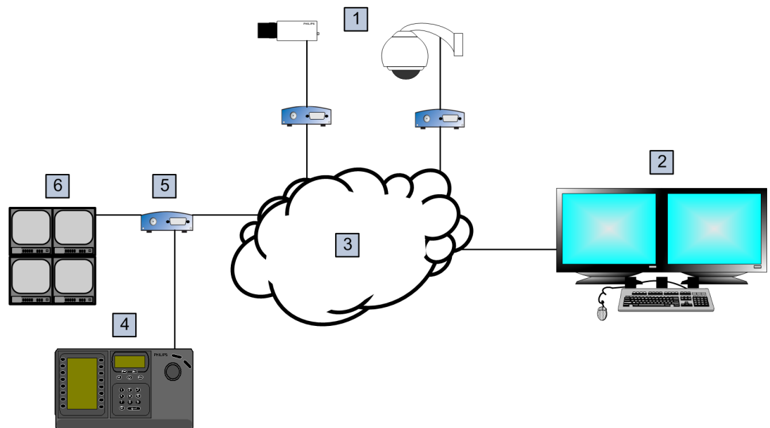
Abbeelding 5.2: Scenario 2: Bosch IntuiKey-bedieningspaneel aangesloten op een decoder
