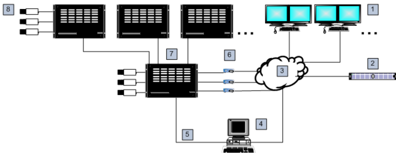
Figura 5.5: Sistema Bosch Allegiant ampliado con matrices satélite
