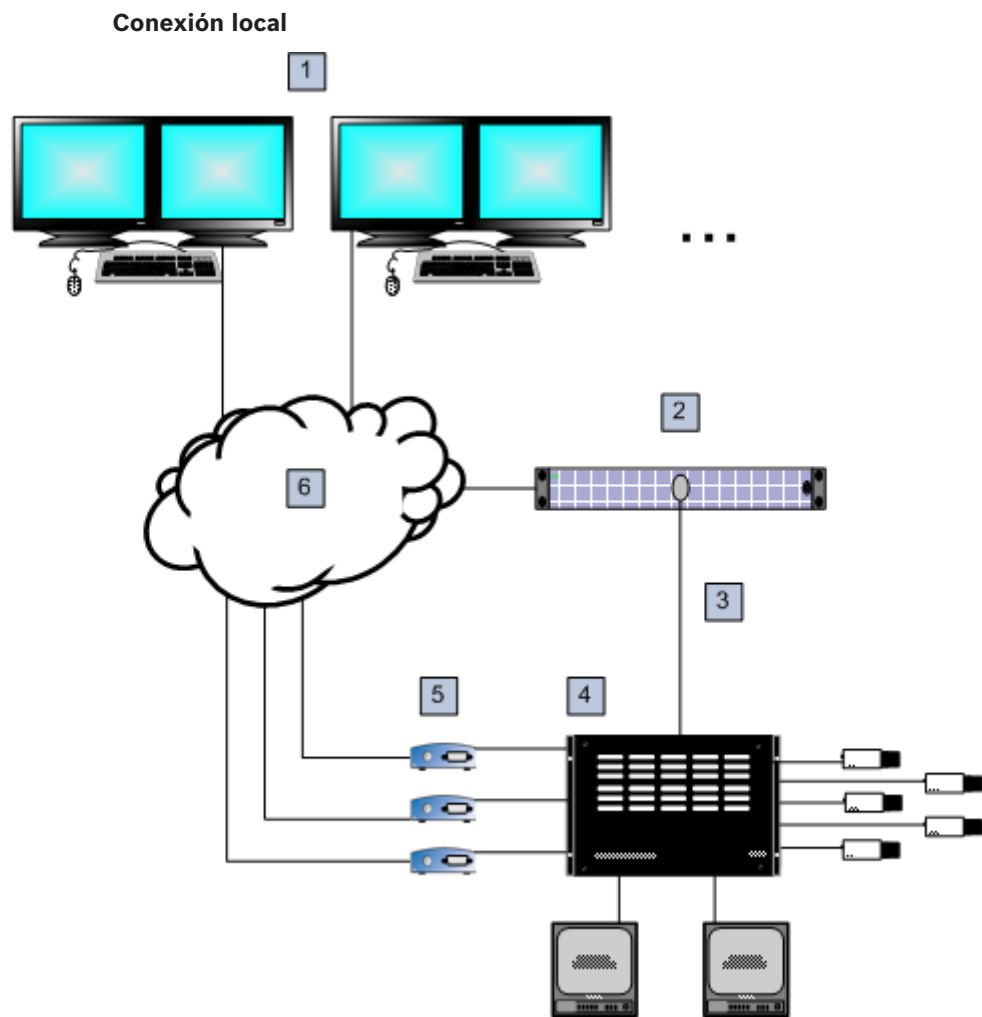
Figura 5.3: Conexión local de Bosch Video Management System a una matriz Allegiant de Bosch
