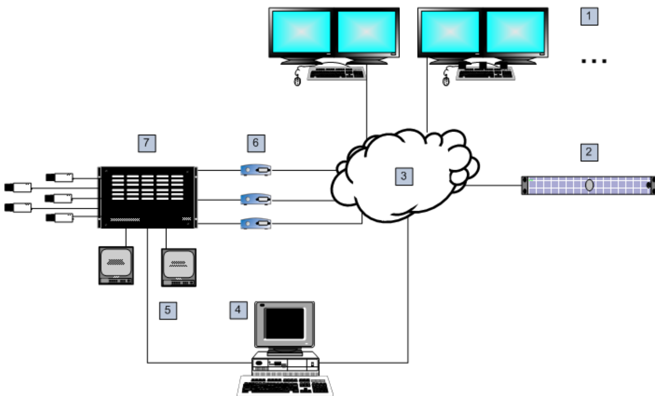
Figura 5.4: Conexión remota de Bosch Video Management System a una matriz Allegiant de Bosch
