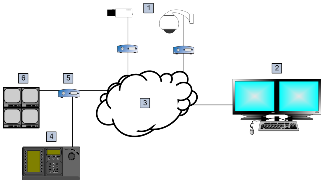
Figura 5.2: Situación 2: teclado IntuiKey de Bosch conectado a un decodificador
